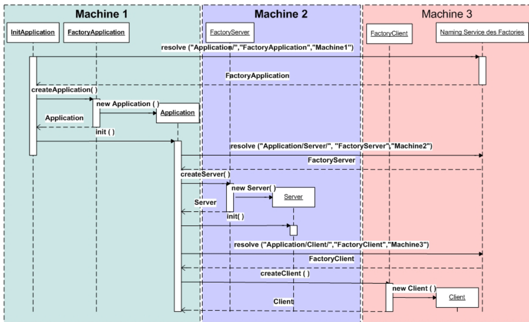
FIG. 3.22 – Création des variables du système par récursivité.
