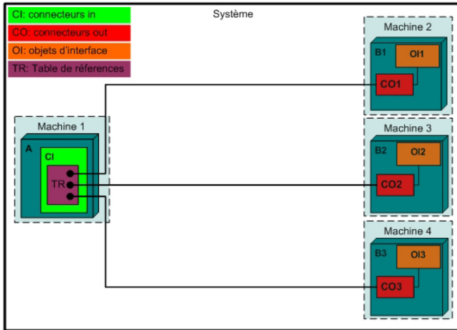
FIG. 3.16 – Connexion manytoone entre deux ensembles d'instances.
