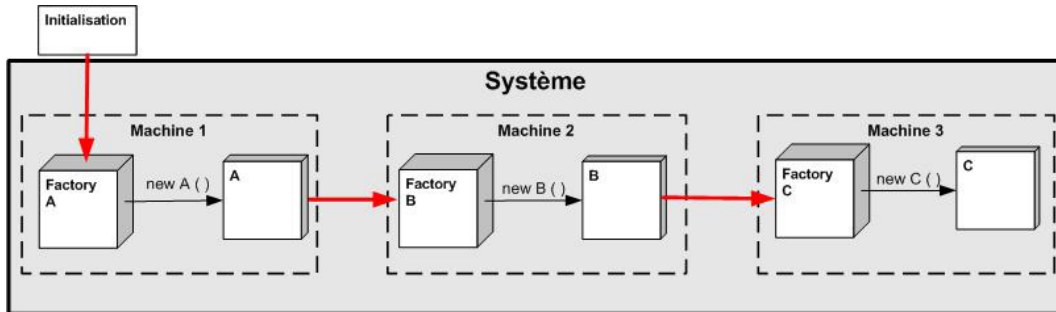
FIG. 3.12 – Déploiement des variables par principe de récursivité.
