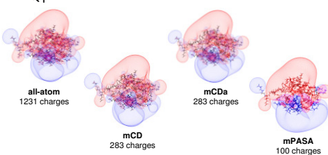
Fig. 5 MEP isocontours of Ubiquitin: -0.05, +0.05 e/bohr.
