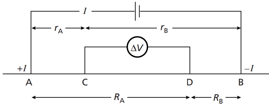
Figure I-13 : Configuration classique d'électrodes utilisée dans les mesures de résistivité électrique (Kearey et al., 2002).
