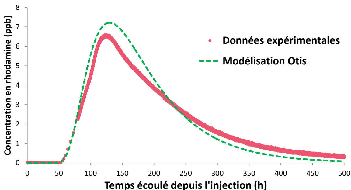
Figure III-26 : Courbe de restitution modélisée et données expérimentales pour le modèle diffusif 4 reches (NUT-TDL).
