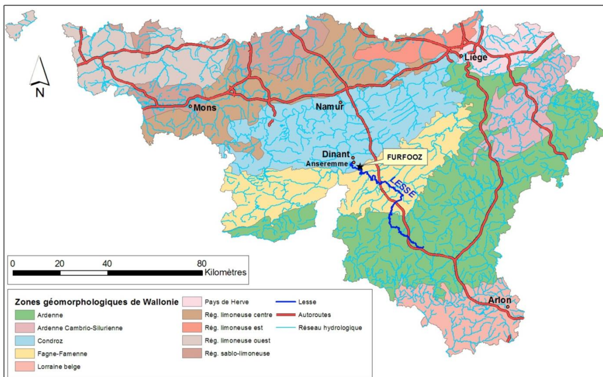
Figure I-1 : Localisation du site de Furfooz sur la carte des zones géomorphologiques de Wallonie.
