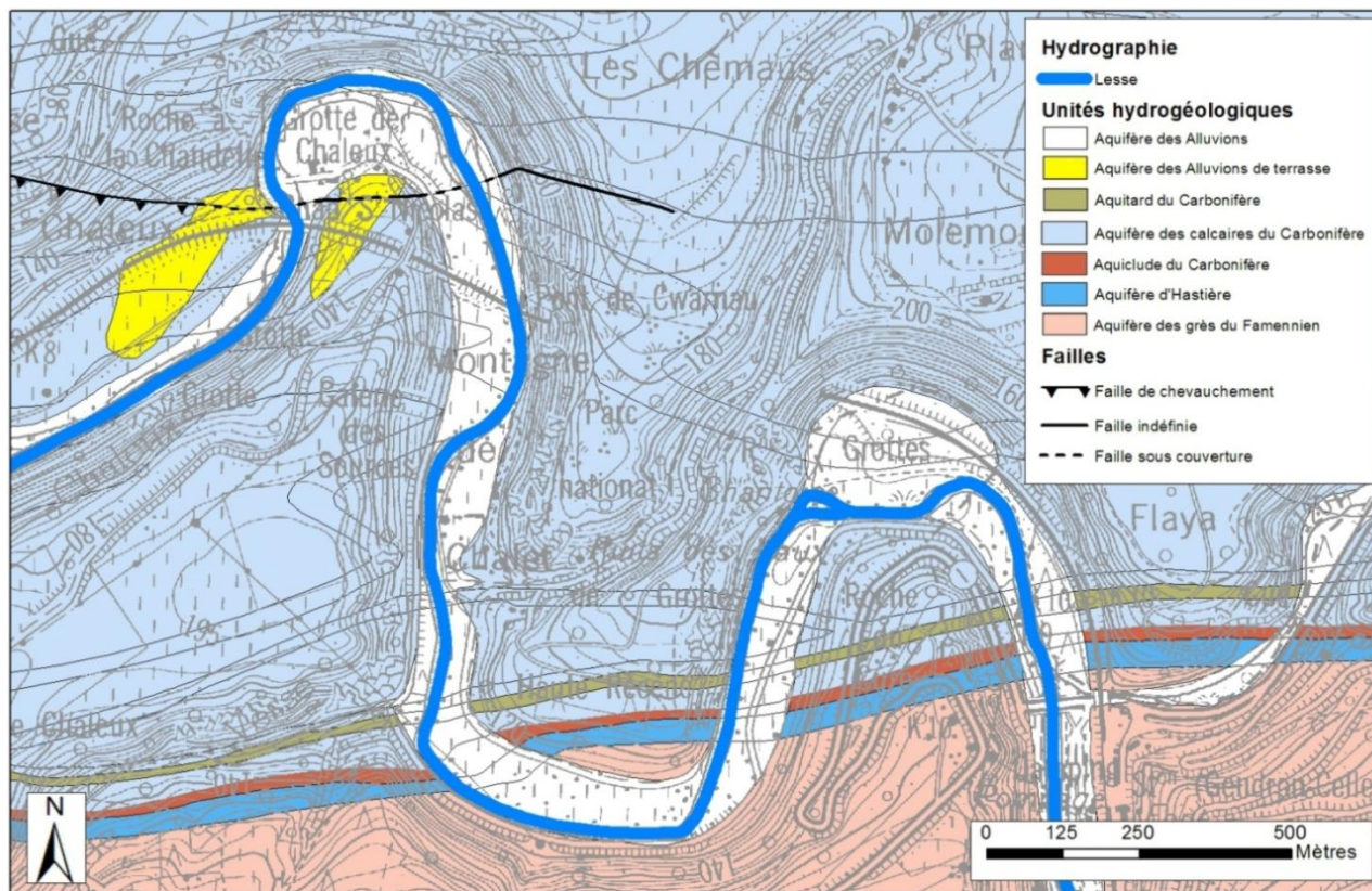
Figure III-2 : Extrait de la carte hydrogéologique de Wallonie Hastière-Dinant (53/7-8) et log stratigraphique reprenant les unités hydrogéologiques affleurantes au sein du massif de Furfooz et leur correspondance géologique (Nogarède et al., 2003 – modifié).
