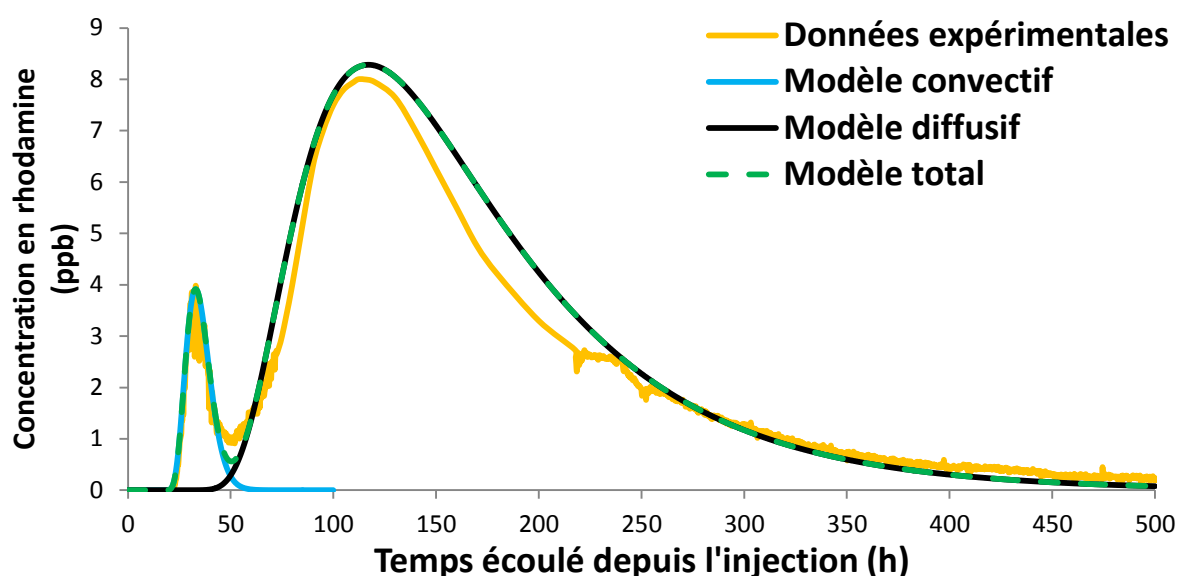
Figure III-29 : Courbes des modèles convectif, diffusif et total comparées aux données expérimentales mesurées à la Galerie des Sources lors du traçage n° 6.
