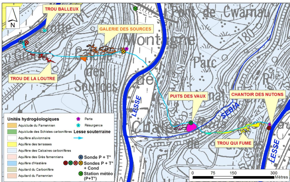
Figure II-1 : Localisation des stations de monitoring dans la zone d'étude – P : Pression, T° : Température, Cond : conductivité électrique.
