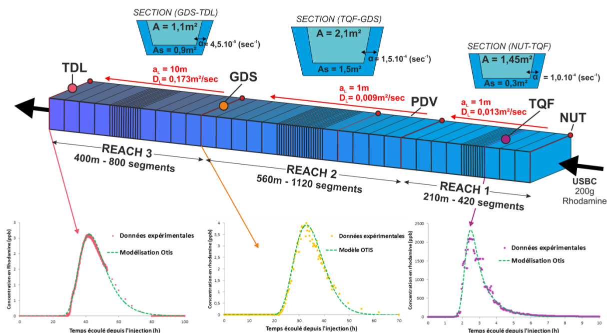
Figure III-21 : Synthèse des résultats de la calibration OTIS du modèle convectif – Pour chaque reach, les paramètres A , A_s , a_L , D_L et \alpha ont été calibrés.
