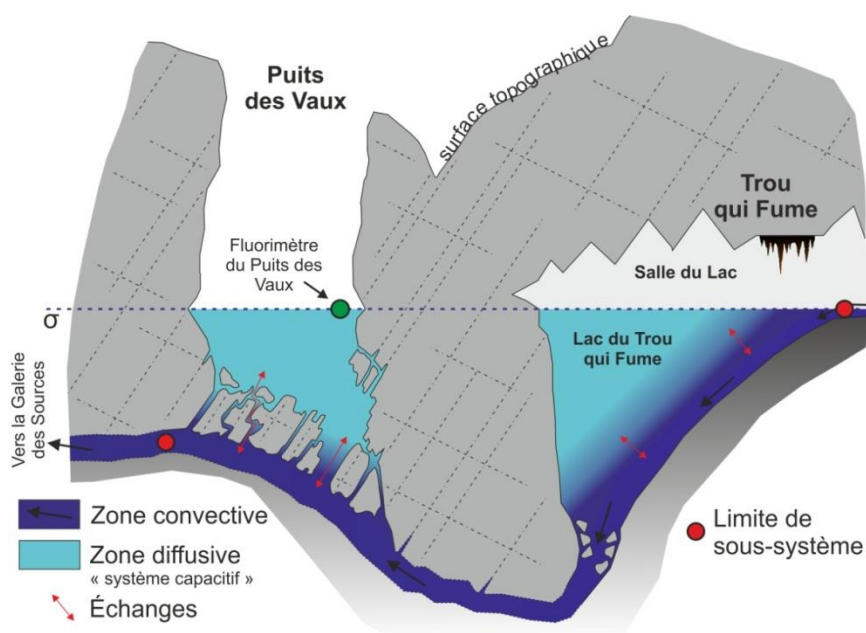
Figure III-14 : Schéma conceptuel du double processus d'écoulement affectant le sous-système de type noyé « Trou qui Fume – Puits des Vaux » (schéma sans échelle).
