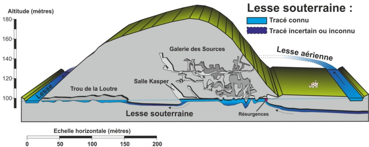
Figure I-7 : Vue schématique du réseau ouest de la Lesse souterraine de Furfooz.
