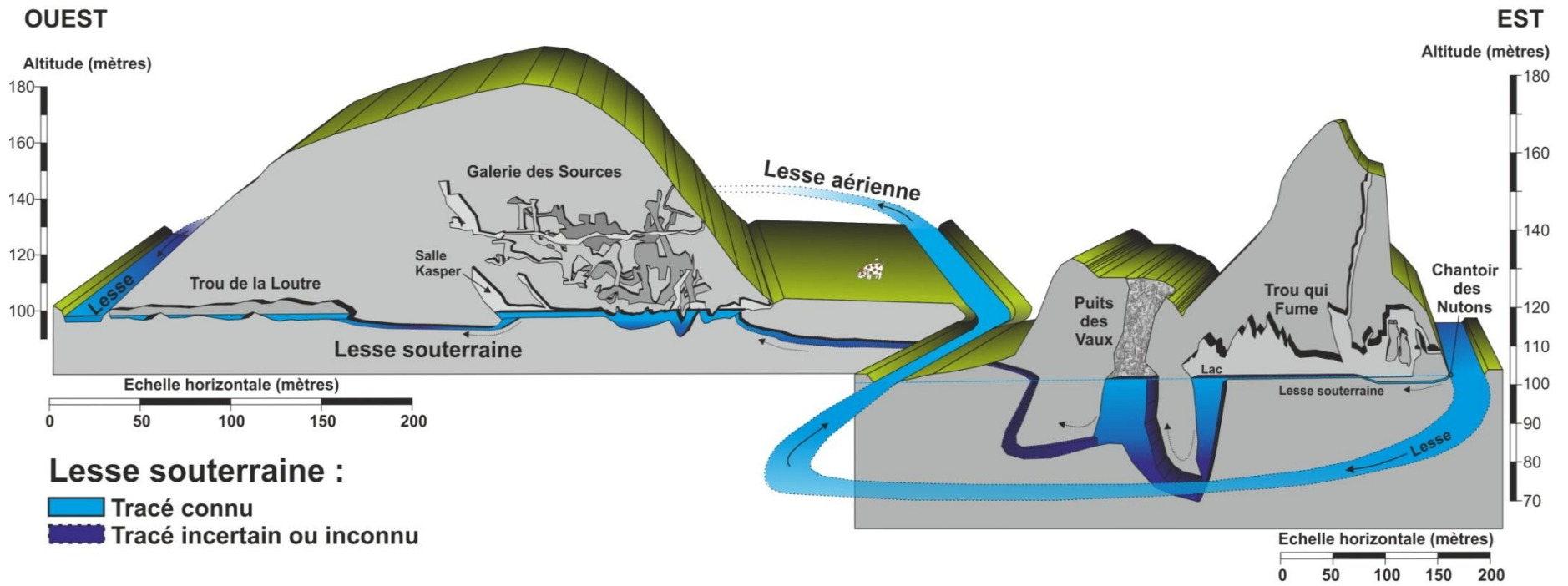
Figure I-10 : Vue en perspective du réseau de la Lesse souterraine de Furfooz.
