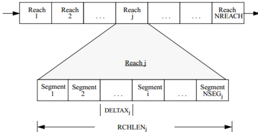
Figure III-9 : Schéma de regroupement de segments en reaches. DELTA_{x_j} : longueur des segments du reach j , RCHLEN_j : longueur du reach j (Runkel, 1998).
