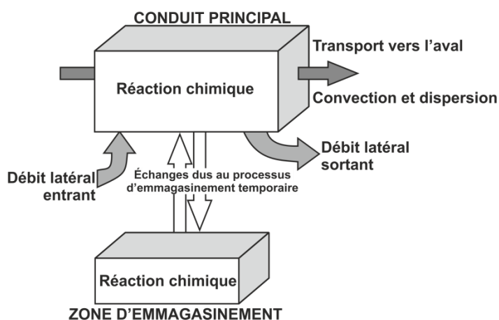
Figure III-6: Modèle conceptuel OTIS montrant les processus affectant le conduit principal et la zone d'emmagasinement (Runkel, 1998 – modifié).
