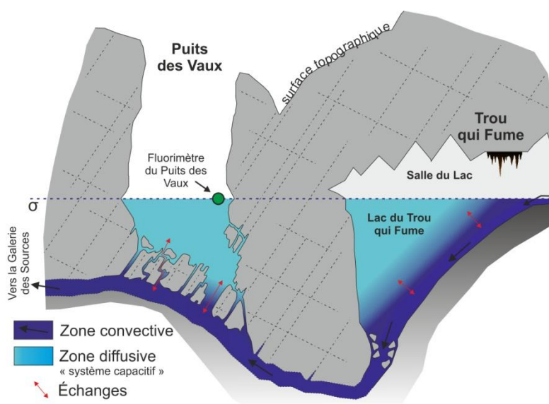
Figure II-11 : Schéma conceptuel du double processus de transport affectant la zone noyée TQF - PDV (schéma sans échelle).
