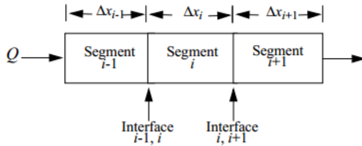
Figure III-8 : Schéma de segmentation et dénomination des différents segments et interfaces (Runkel, 1998).
