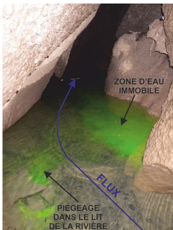
Figure III-5 : Illustration du phénomène d'emménagement temporaire lors d'une injection d'uranine à la Galerie des Sources.
