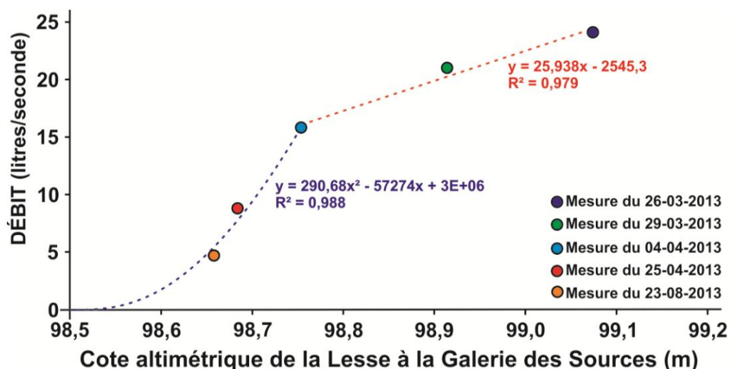
Figure II-4 : Courbe de tarage à la station de la Galerie des Sources.
