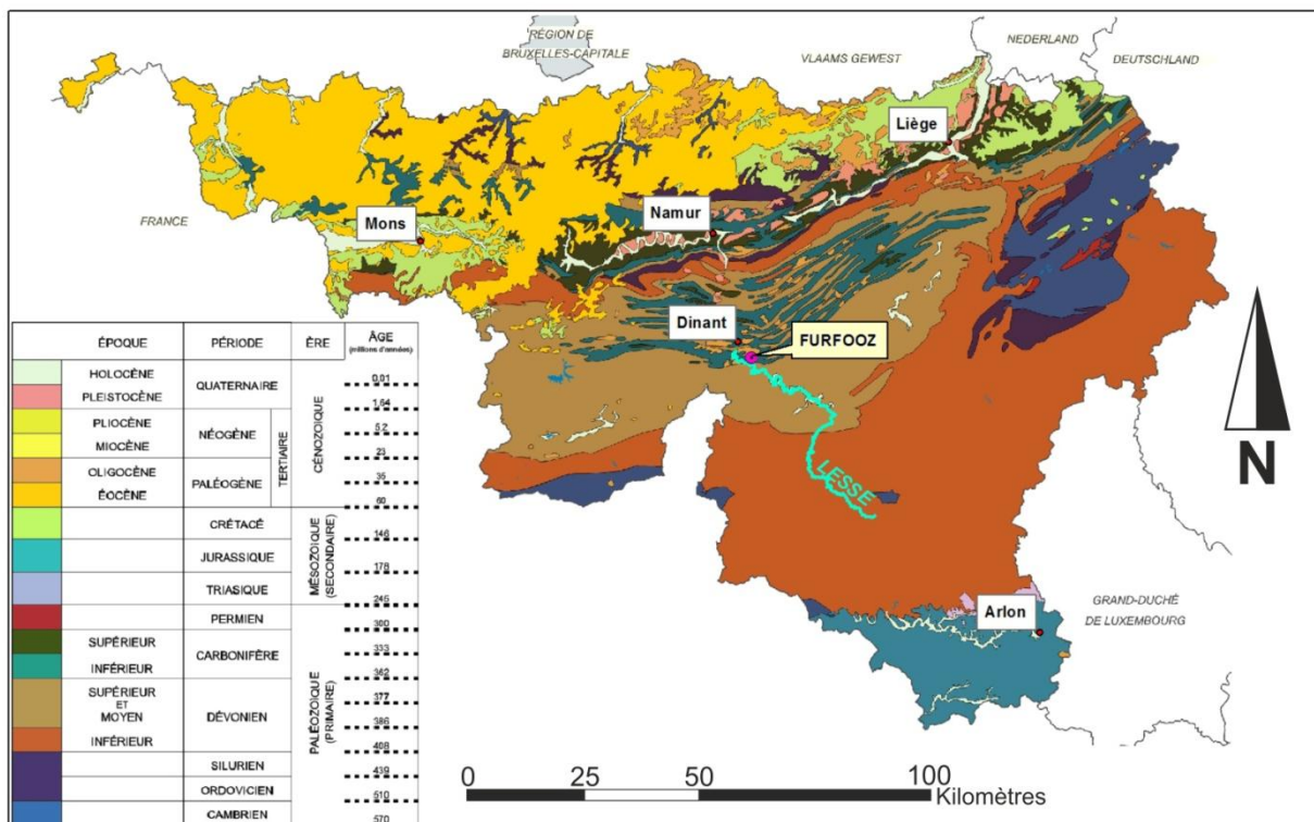
Figure II-1 : Localisation du site d'étude sur la carte géologique de Wallonie (de Béthune, 1961).
