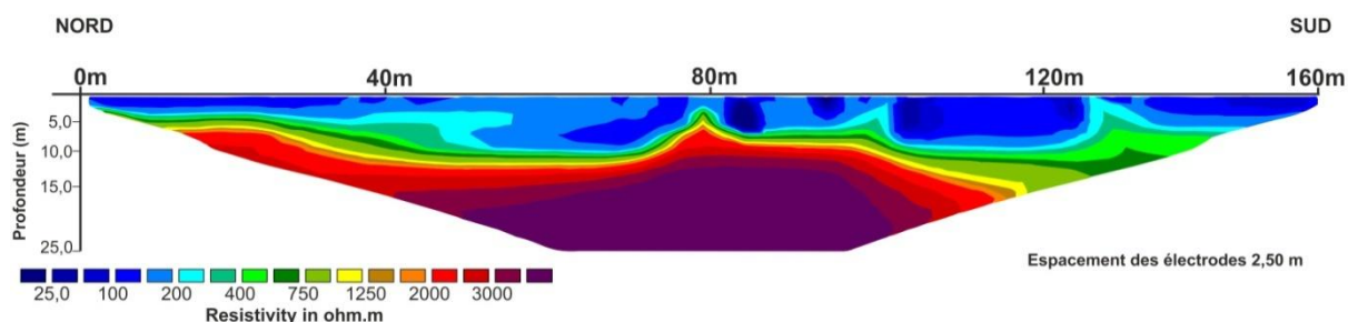
Figure I-16 : Profil de tomographie électrique n°2.
