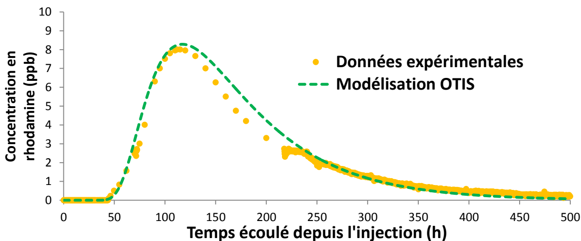
Figure III-25 : Courbe de restitution modélisée et données expérimentales pour les reaches 1 à 3 (NUT-GDS).
