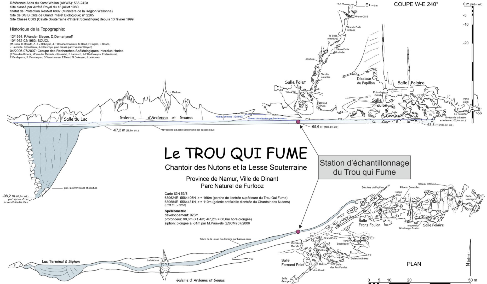
Figure I-6 : Topographie du Trou qui Fume (Groupe des recherches spéléologiques interclub Hadès, 2007).
