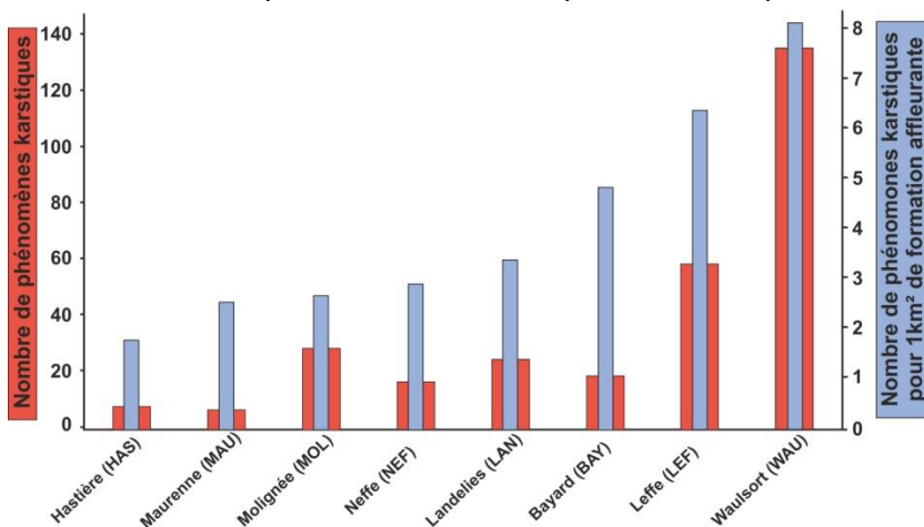
Figure I-6 : Répartition des phénomènes karstiques entre les formations carbonatées de la région de Furfooz (De Schepper, 2007).
