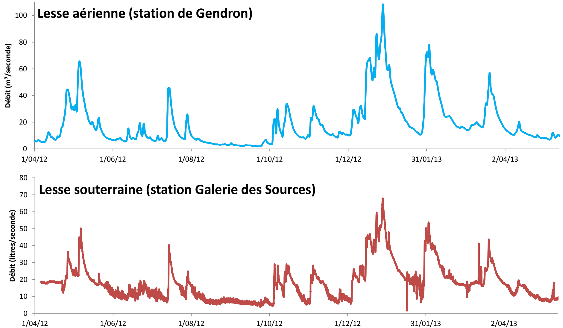
Figure II-5 : Chroniques de débits pour la Lesse aérienne (Gendron) et la Lesse souterraine (Galerie des Sources) – Noter la différence d'unité des axes verticaux.
