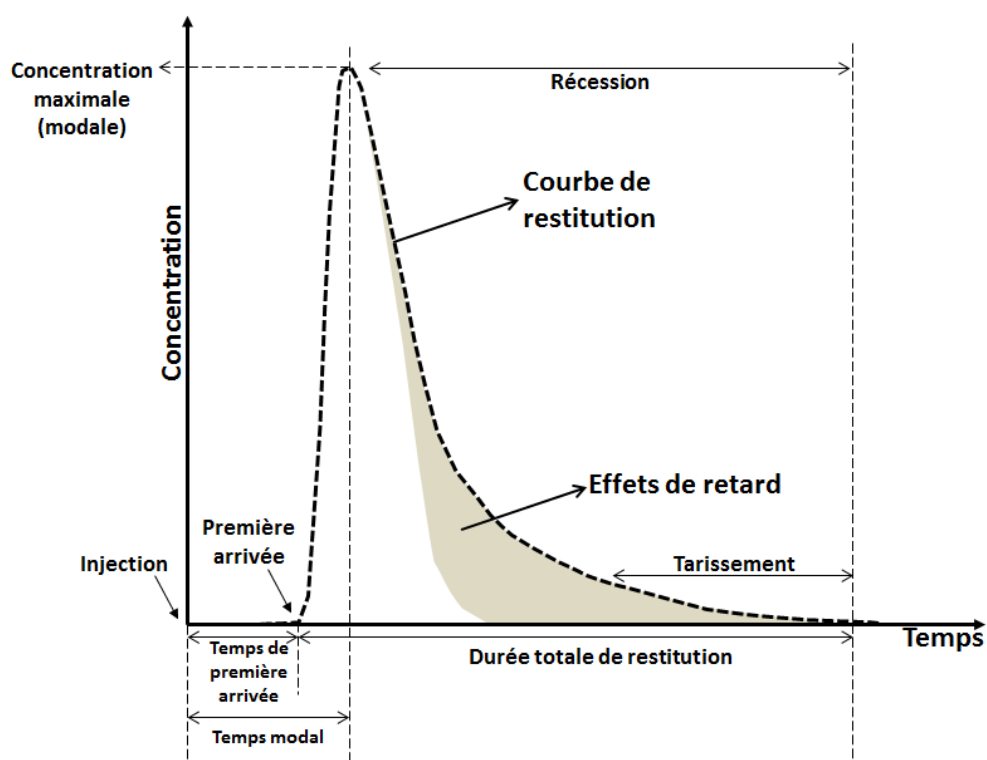
Figure II-1 : Exemple de courbe de restitution et des informations qui y figurent (Bonniver, 2011 – modifié).
