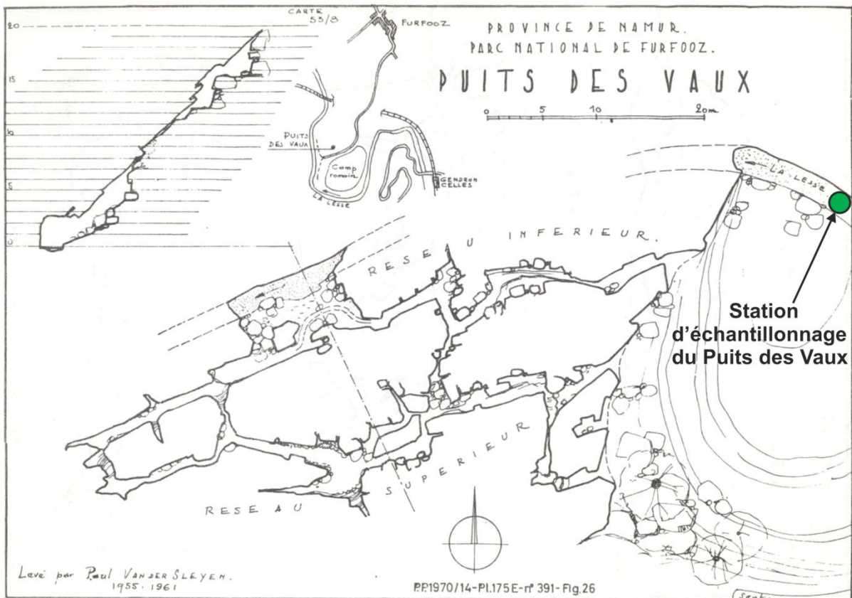
Figure I-5 : Topographie du Puits des Vaux (Van der Sleyen, 1961).
