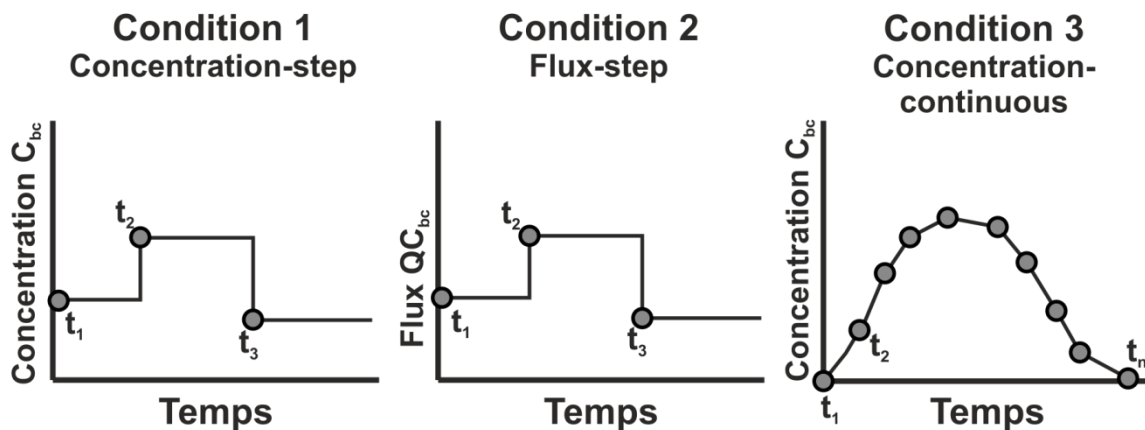
Figure III-11 : Différents types de conditions limite amont - C_{bc} : Concentration à l'entrée du modèle au temps i , t_i : temps de mise à jour de la concentration à l'entrée du système, imposé par l'utilisateur (Runkel, 1998 – modifié).
