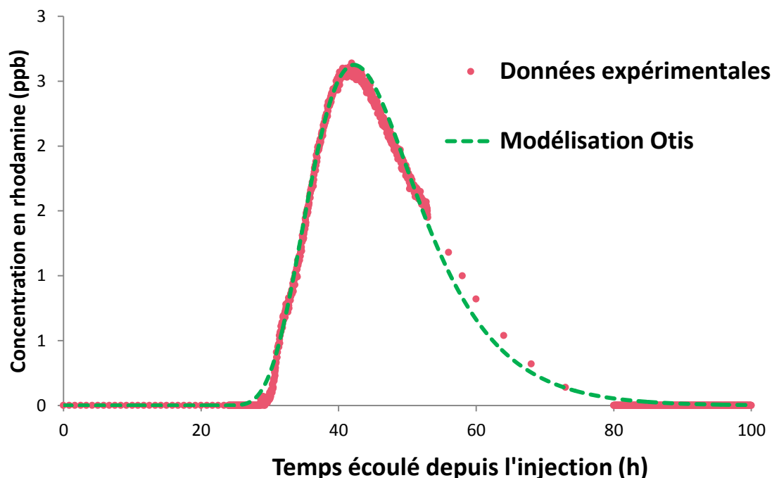
Figure III-20 : Courbe de restitution modélisée et données expérimentales pour l'ensemble du modèle convectif 3 reaches (NUT-TDL).
