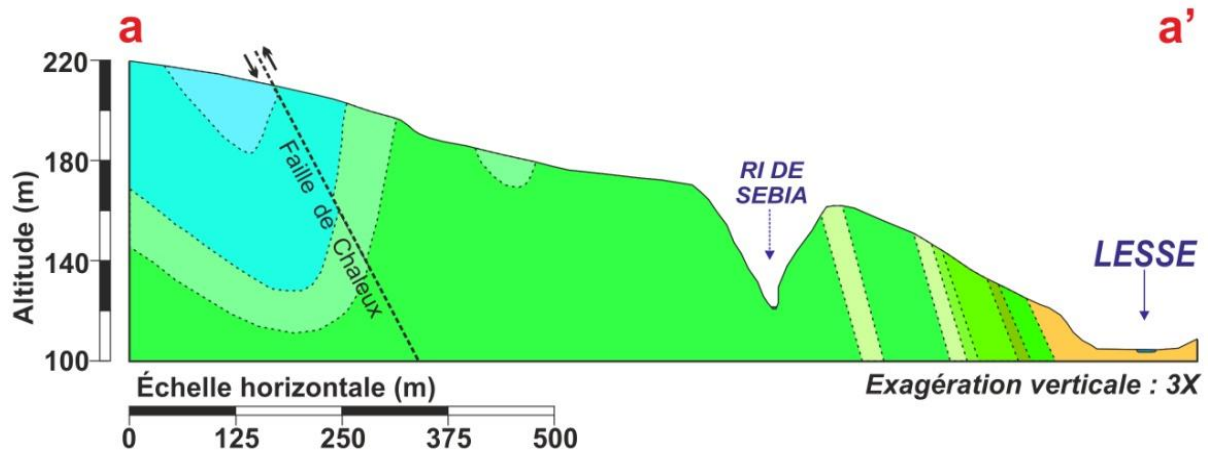
Figure II-7 : Coupe géologique a-a' au travers du massif de Furfooz.
