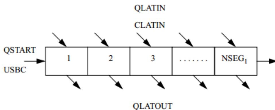
Figure III-7: Subdivision du système conceptuel en N segments et inputs du modèle – QSTART : débit à l'amont du système, USBC : conditions d'introduction du soluté dans le modèle, QLATIN : débit latéral entrant, CLATIN : Concentration du soluté entrant, QLATOUT : débit latéral sortant (Runkel, 1998).
