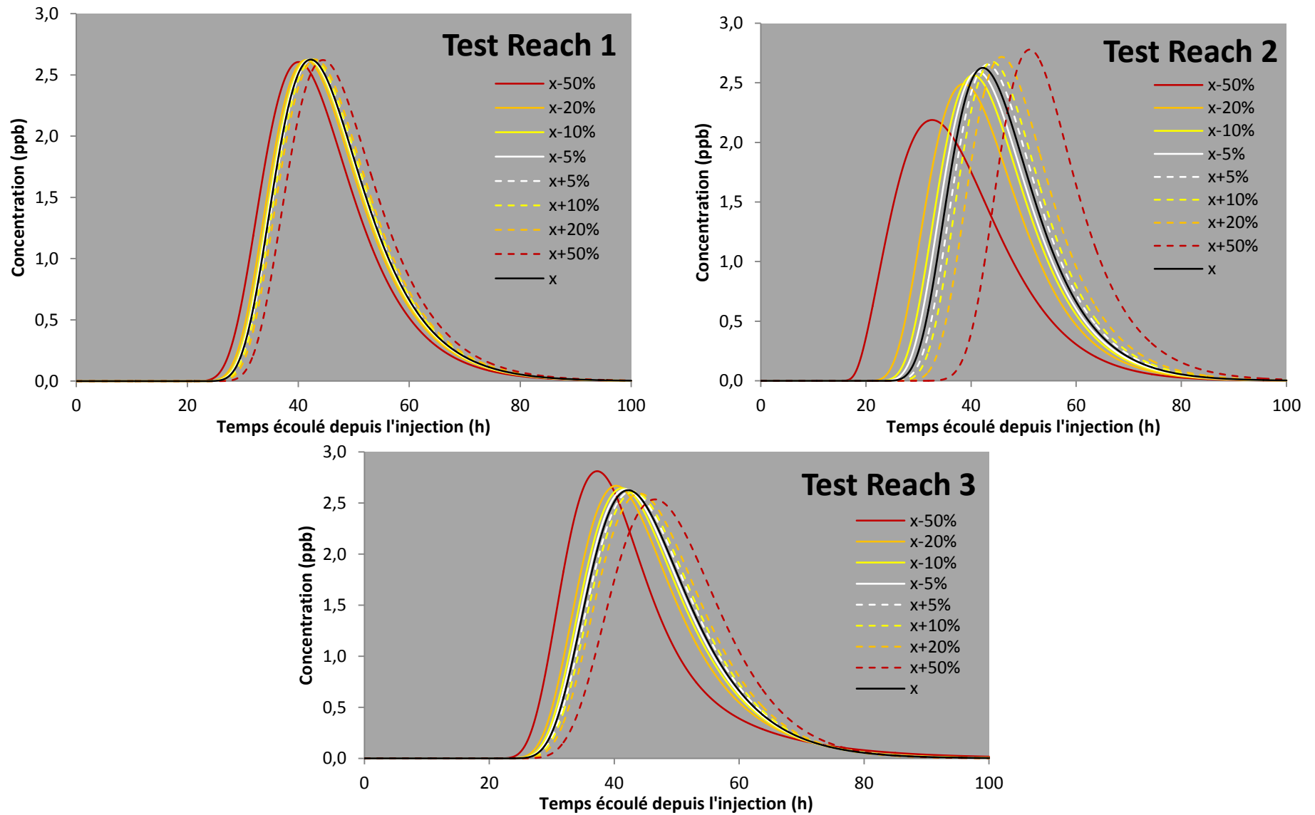
Figure III-23 : Courbes modélisées des tests de sensibilité du paramètre A pour les différents reaches du modèle convectif.
