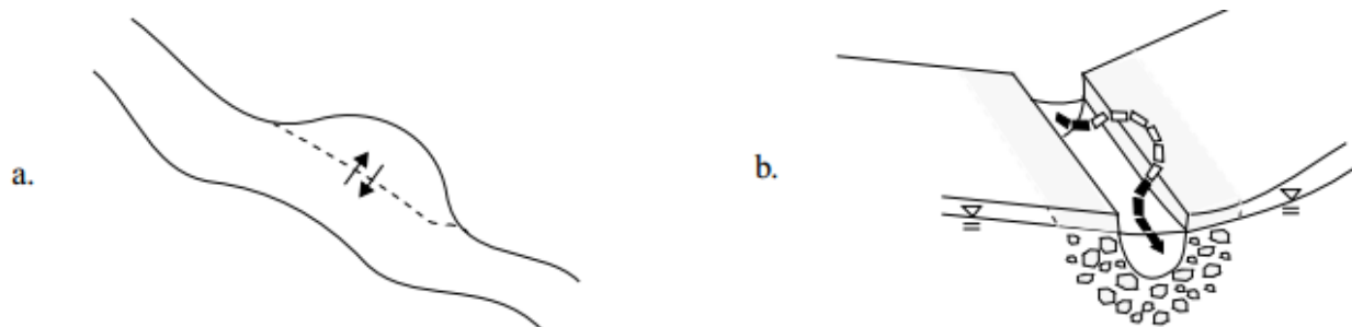
Figure III-4: Processus d'emménagement temporaire – a : volumes d'eau peu mobile, b : piégeage dans le milieu poreux formant le lit et les rives de la rivière. Les flèches montrent les mouvements de soluté entre la zone d'écoulement principal et les zones d'emménagement temporaire (Runkel, 1998).
