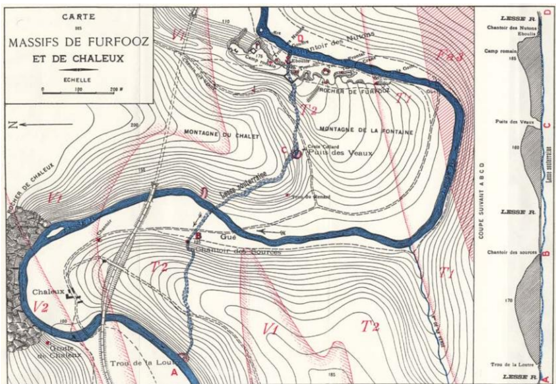
Figure I-1 : La double boucle de la Lesse, à Furfooz, traversée par la Rivière souterraine (Vandebroek et al., 1910).
