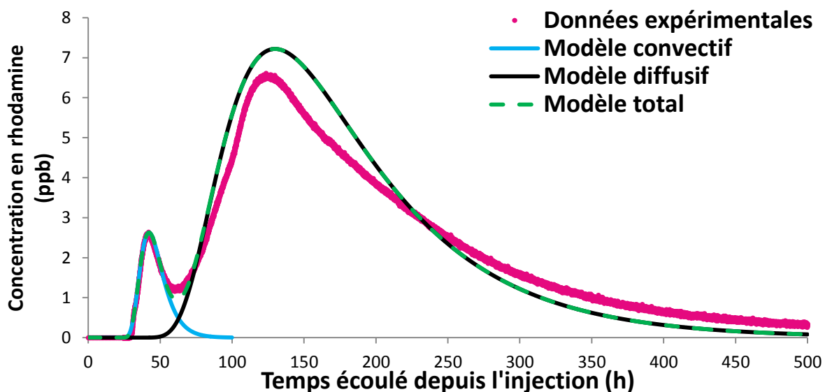
Figure III-30 : Courbes des modèles convectif, diffusif et total comparées aux données expérimentales mesurées au Trou de la Loutre lors du traçage n° 6.
