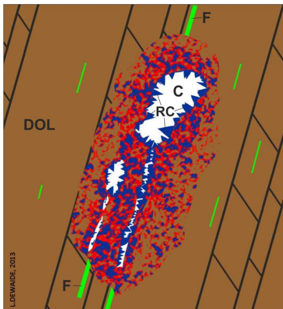
Figure I-7 : Schéma type des phénomènes karstiques développés dans le waulsortien – C : cavité, DOL : encaissant dolomitique, RC : rhomboèdres de calcite, F : faille, couleur rouge : dolomie dédolomitisée, couleur bleue : calcite (Dewaide et al., soumis).
