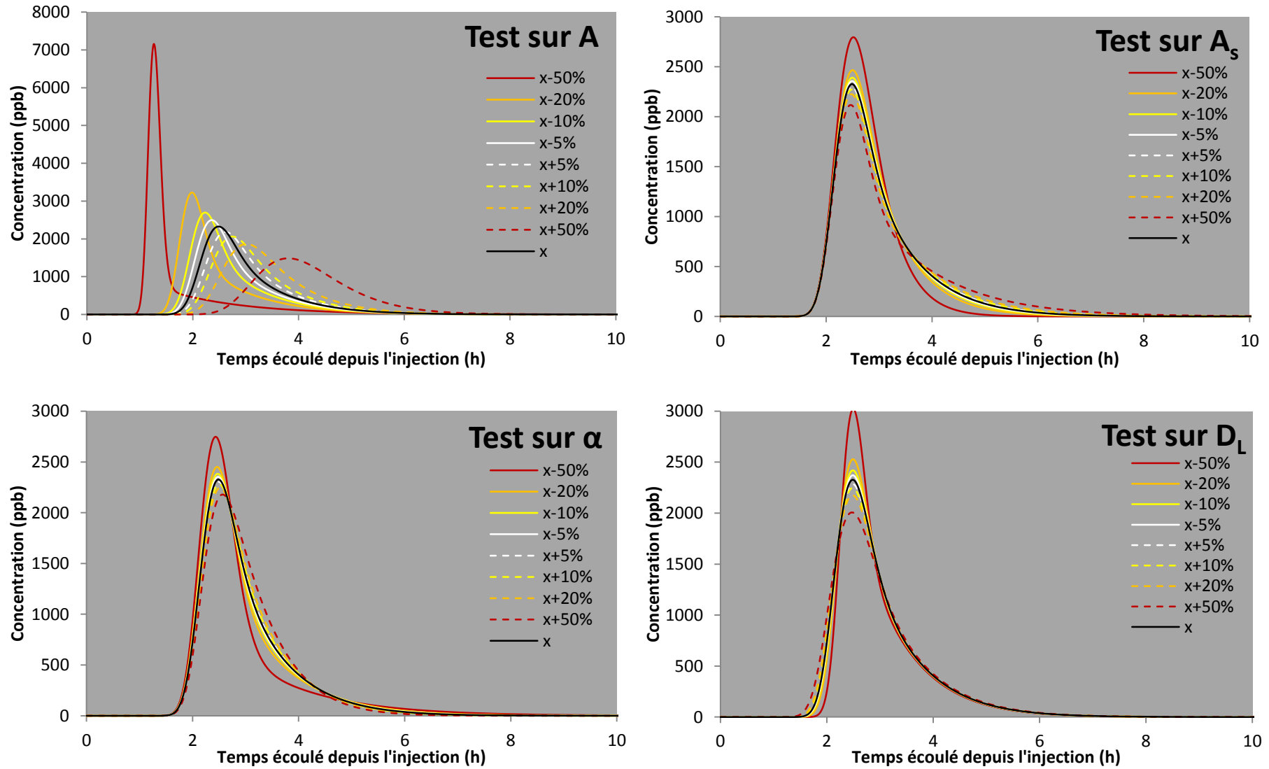
Figure III-22 : Courbes modélisées des tests de sensibilité pour A , A_s , D_L et \alpha (Modèle convectif – reach 1).
