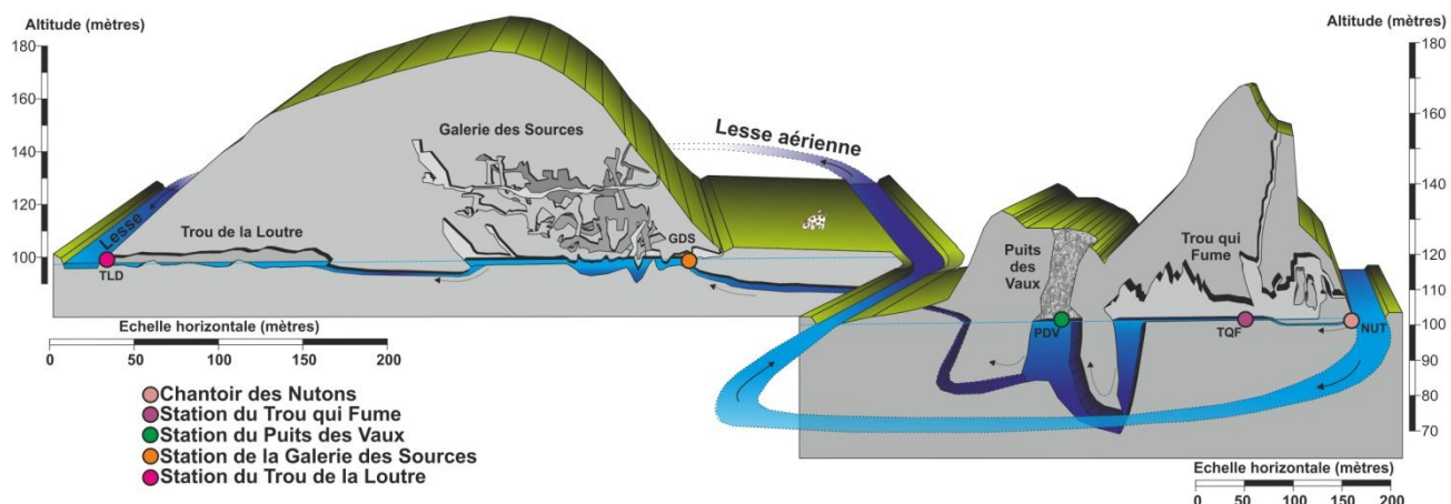
Figure II-4 : Localisation des différentes stations utilisées lors des 9 essais de traçage quantitatifs.
