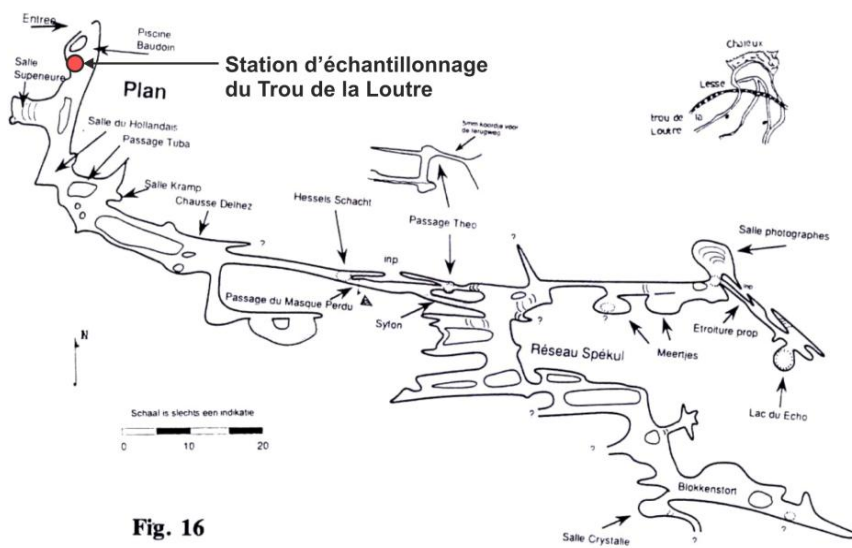
Figure I-7 : Vue schématique du réseau ouest de la Lesse souterraine de Furfooz.
