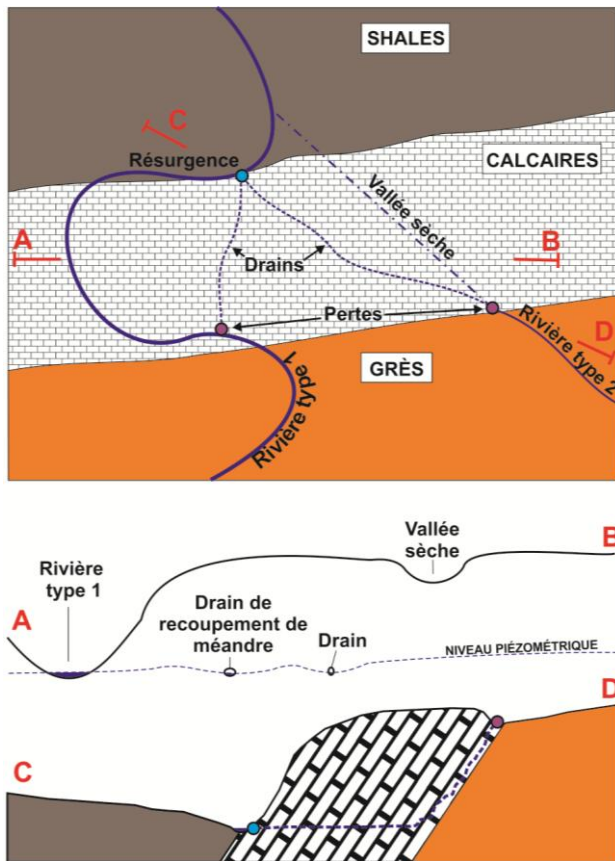
Figure 1-5 : Les différents réseaux karstiques en Belgique (Quinif, 1977 – modifié).
