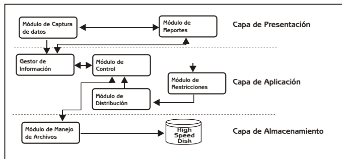
Figura 1. Diagrama de la Arquitectura de CREAR
