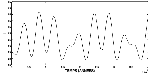
FIGURE 4.18 – Graphique de l'évolution temporelle de i pour le problème des trois corps étudié dans l'article [1] avec l'erreur dans le coefficient C_3 et une inclinaison i = 15^\circ .
