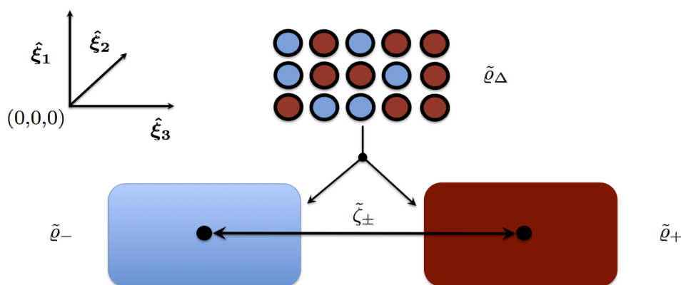
FIGURE III.2.7 – Illustration de la métrique \tilde{\zeta}_{\pm} , obtenue à partir des densités \tilde{\rho}_{\pm} .
