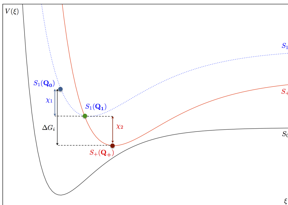
FIGURE VI.1.4 – Profil énergétique – Transfert de charge non-activé.
