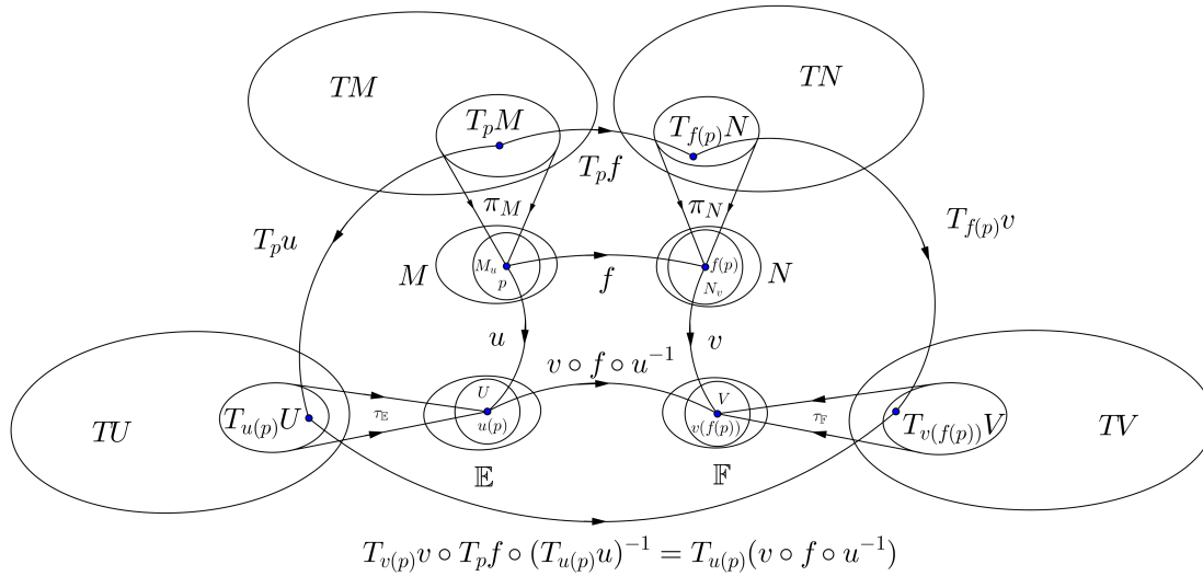
FIGURE 3.2: Tangentielle et sa représentation en coordonnées
