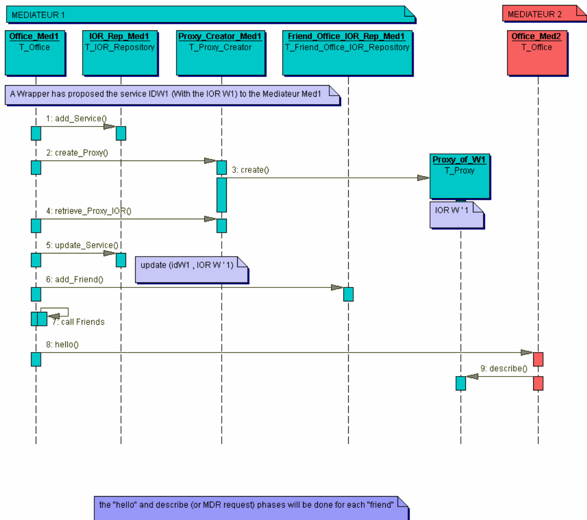
Figure 22 : Sequence diagram illustrant la communication des services entre médiateurs
