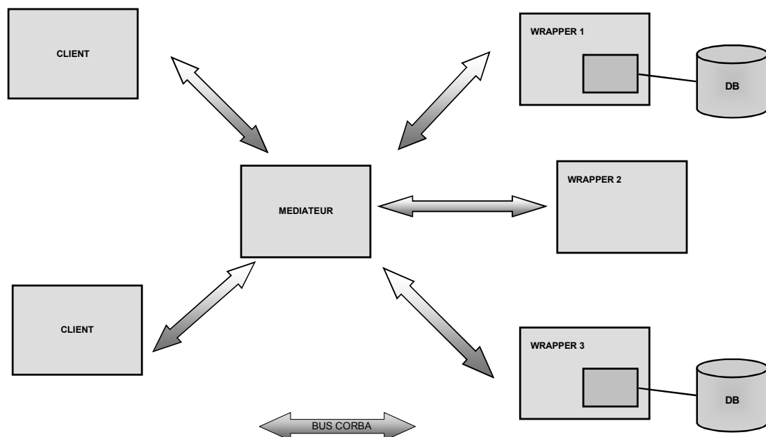
Figure 15 : Architecture générale à un médiateur
