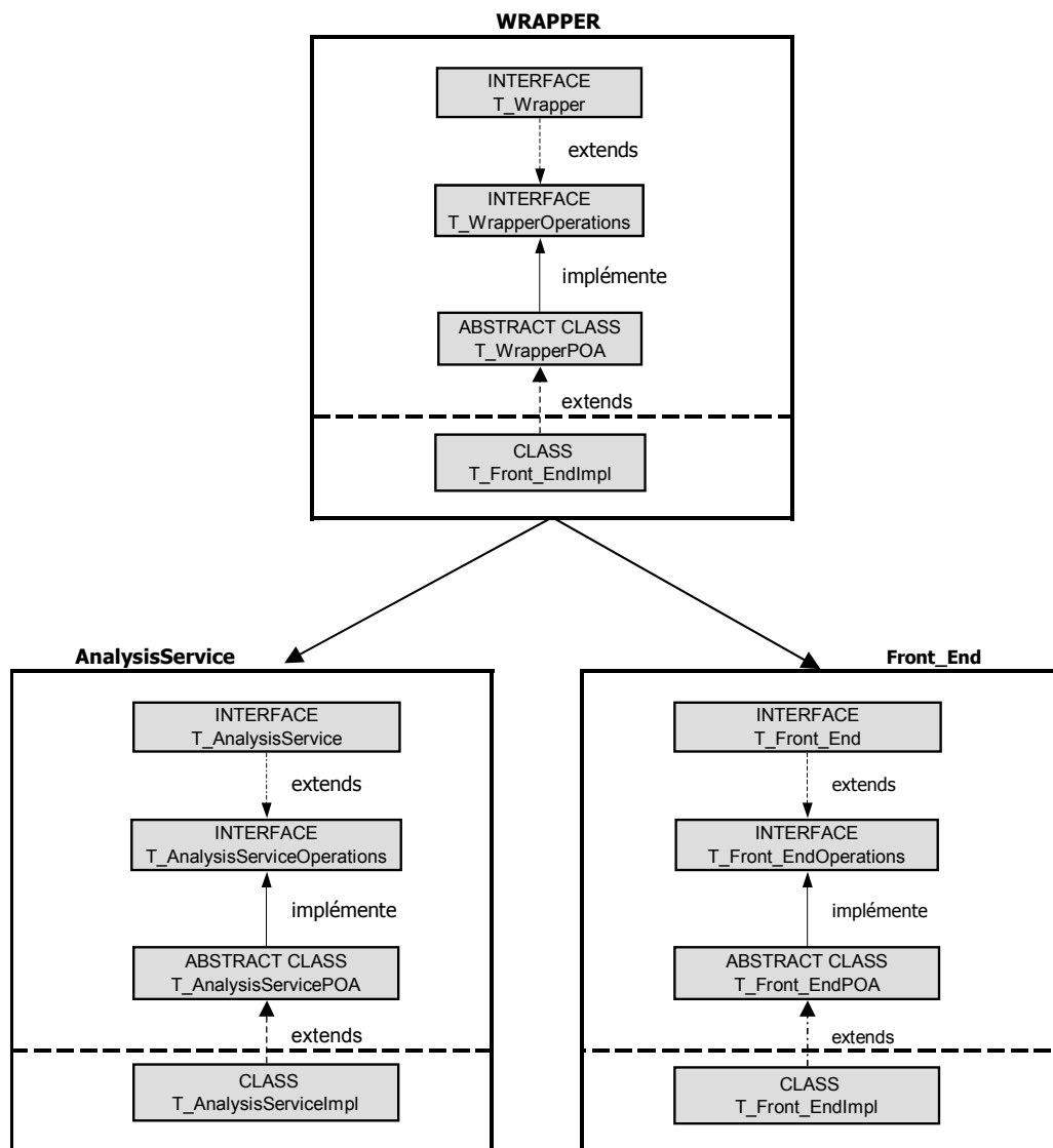
Figure 29 : Structure d'un wrapper (2)
