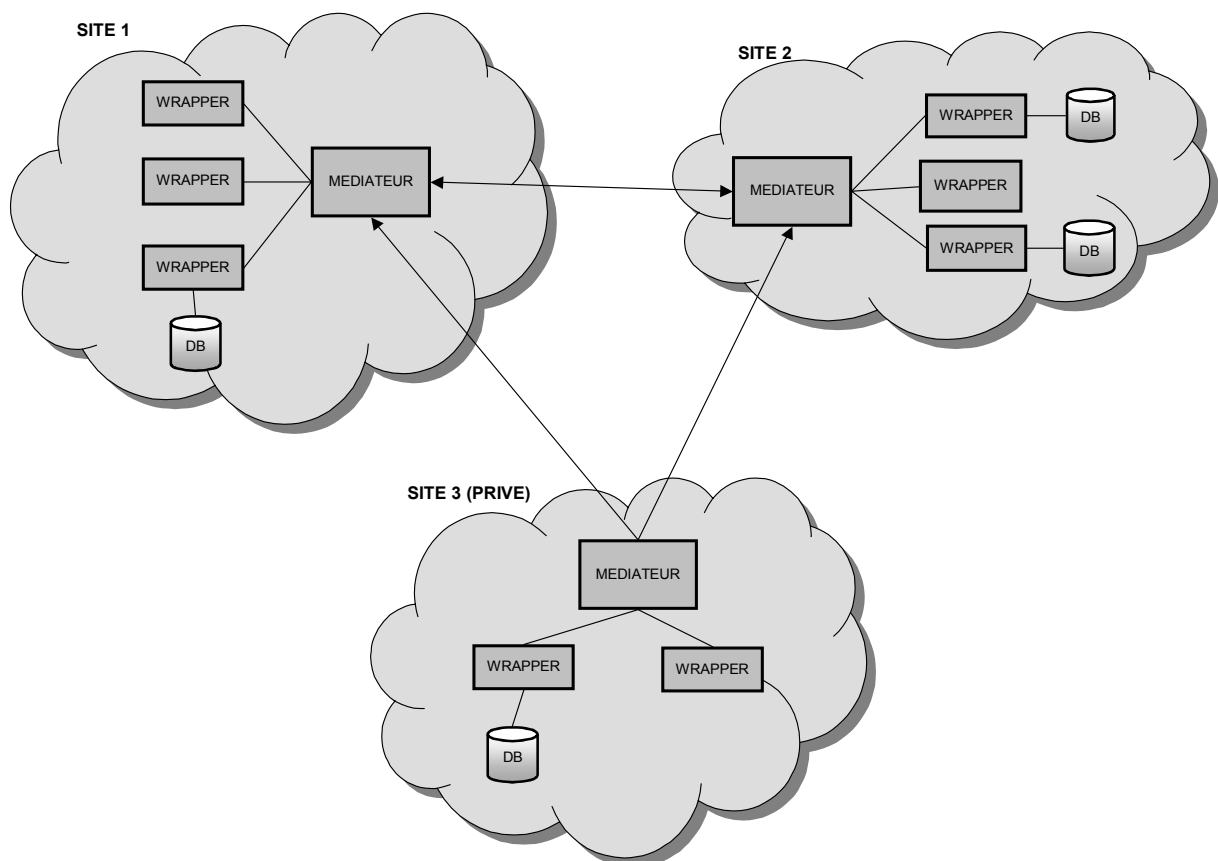
Figure 21 : Architecture générale à plusieurs médiateurs
