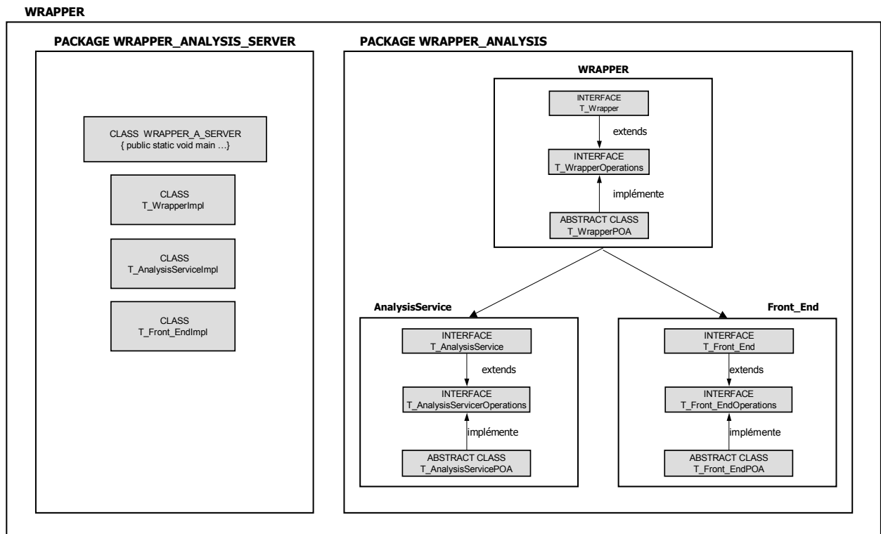
Figure 30 : Vue complète du déploiement d'un wrapper
