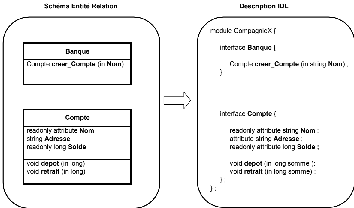
Figure 9 : Exemple d'application définie en IDL
