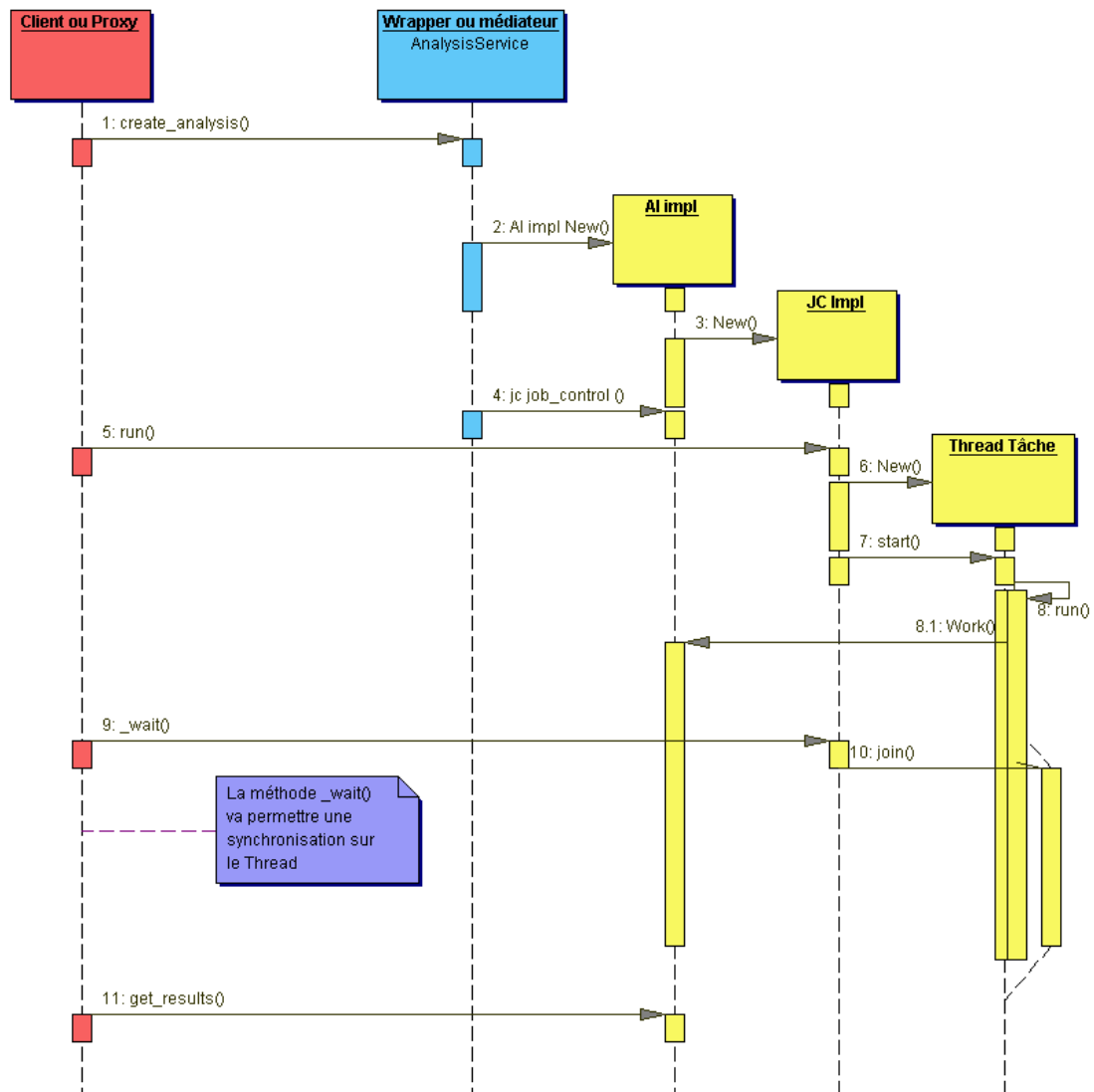
Figure 31 : Sequence diagram illustrant l'implémentation du create_analysis()
