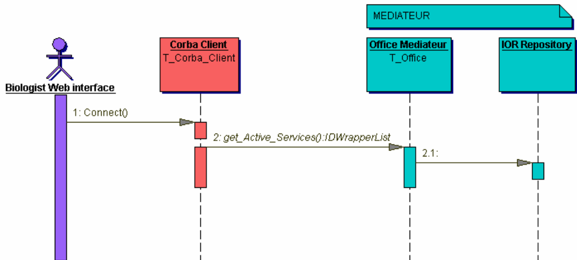
Figure 17 : Sequence diagram illustrant la recherche des services actifs
