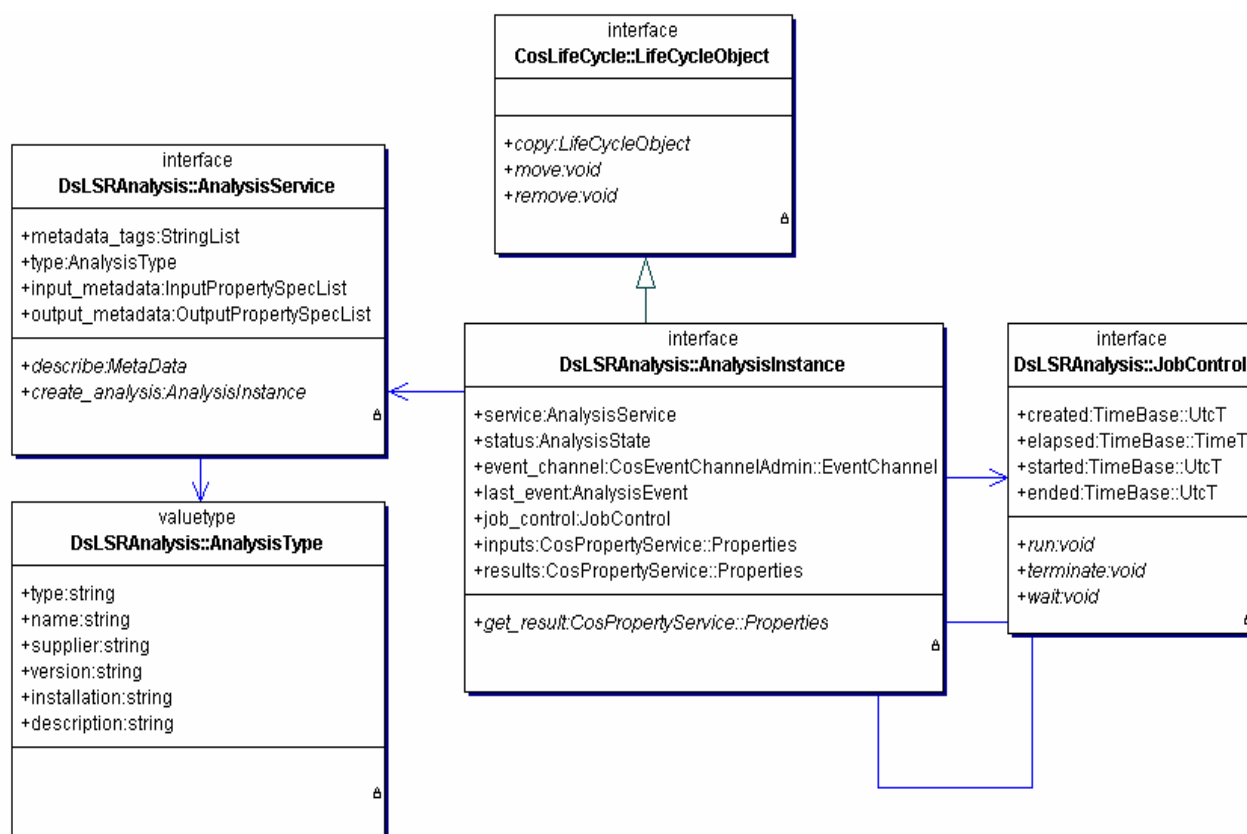
Figure 12 : Principales Interfaces du module DsLSRAnalysis
