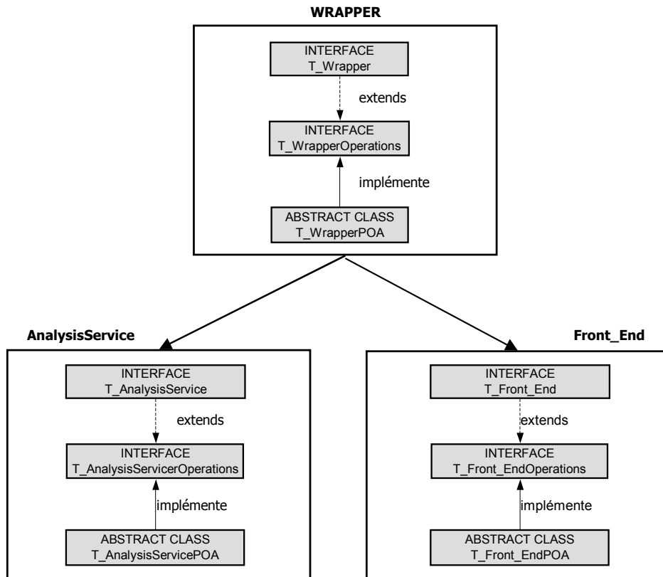
Figure 28 : Structure d'un wrapper (1)
