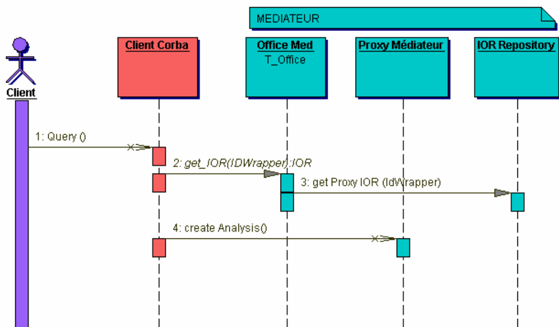
Figure 19 : Sequence diagram illustrant une demande d'analyse au médiateur
