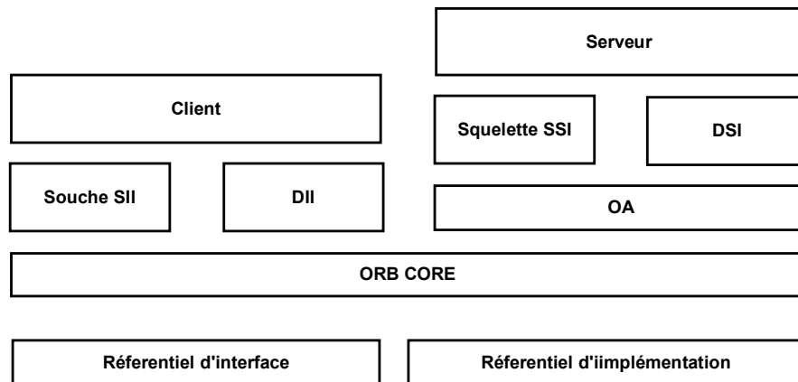
Figure 10 : Vue de l'architecture
