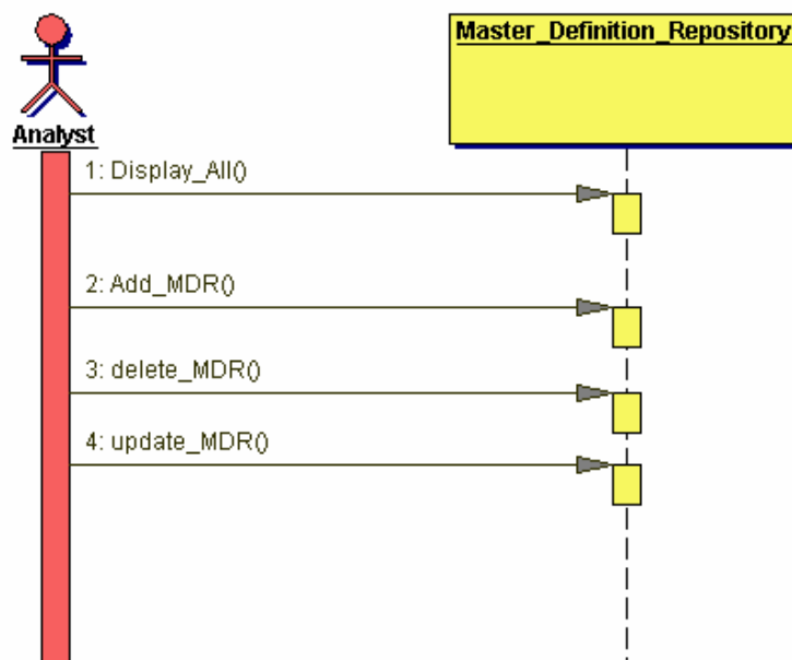
Figure 18 : Sequence diagram schématisant le fonctionnement du MDR
