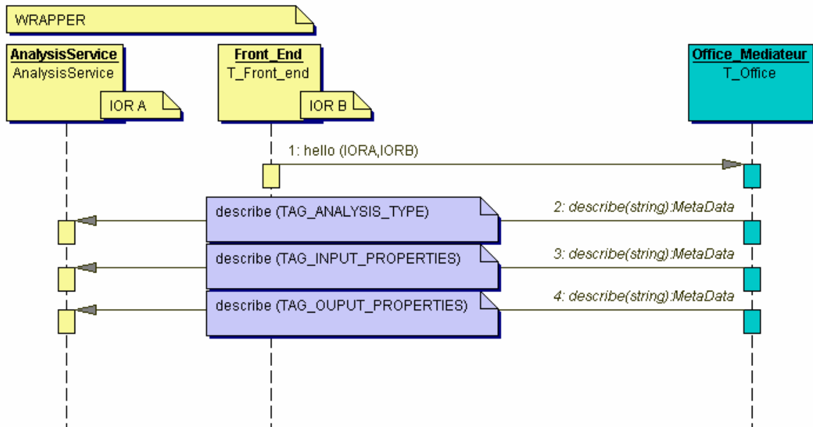
Figure 16 : Sequence diagram illustrant la déclaration d'un wrapper au médiateur
