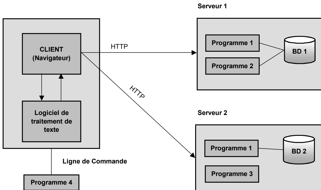
Figure 14 : Représentation de la situation actuelle
