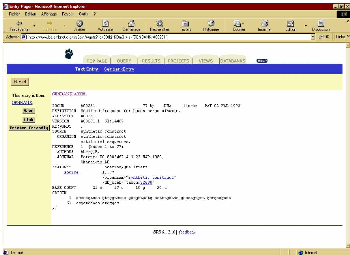
Figure 5 : Récupération d'une entrée avec SRS
