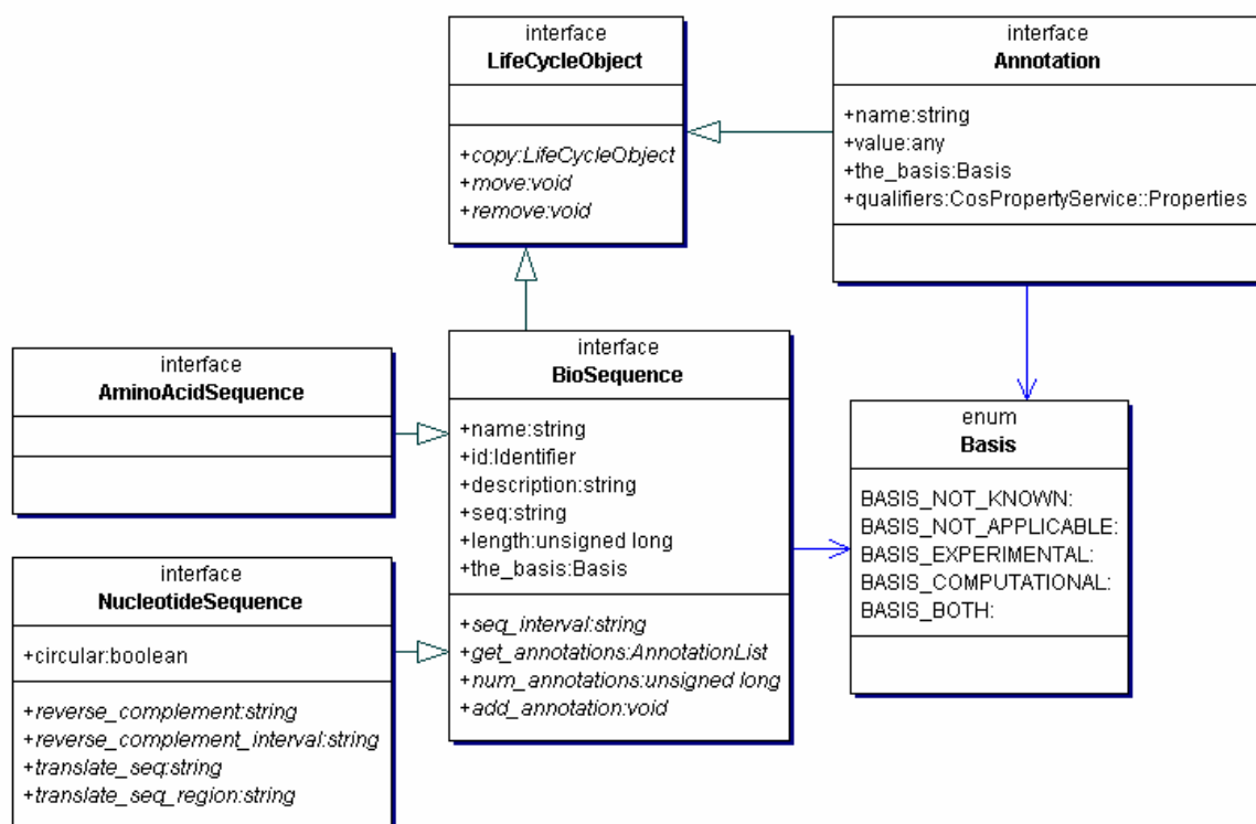
Figure 11 : Principales Interfaces du module DsLSRBioObjects
