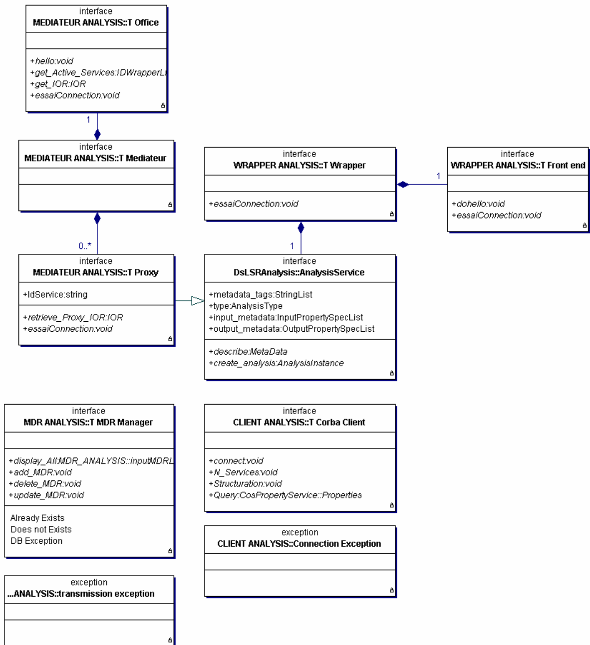
Figure 27 : Class diagram des éléments propres à notre architecture
