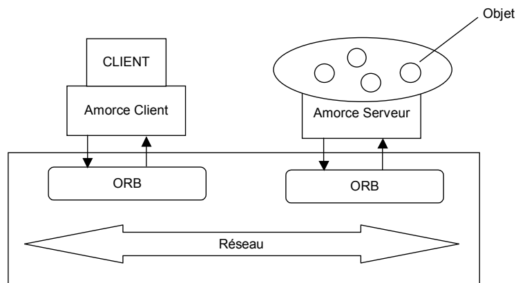
Figure 8 : Le modèle CORBA
