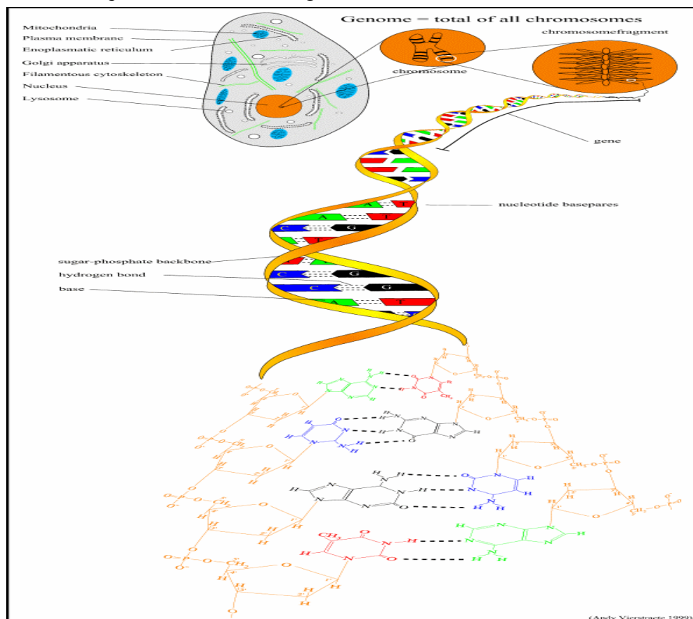
Figure 1 1 : l'ADN
