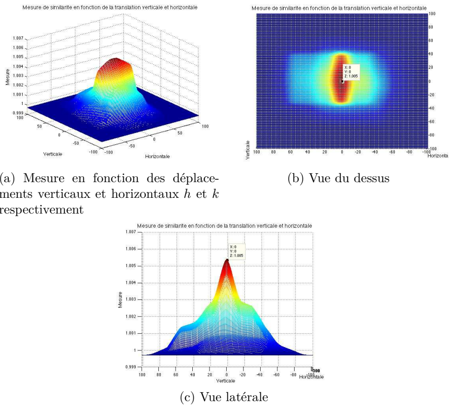
FIGURE 2.21 – Mesure de similarité (SSIM) en fonction des paramètres de translation.
