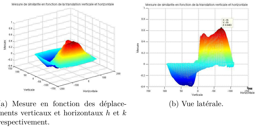
FIGURE 2.11 – Mesure de similarité (coefficient de Pearson) en fonction des paramètres de translation.
