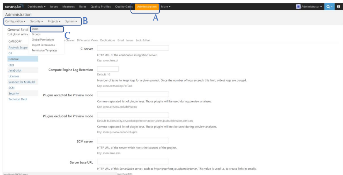
Figure 24: SonarQube – Administration. Groupe A : Item de menu permettant d'accéder à la page. Groupe B : sous-menu de la fonctionnalité « Administration ». Groupe C : Item de sous-menu « Security > Users » permettant d'accéder à la gestion des utilisateurs de l'instance courante de SonarQube.
