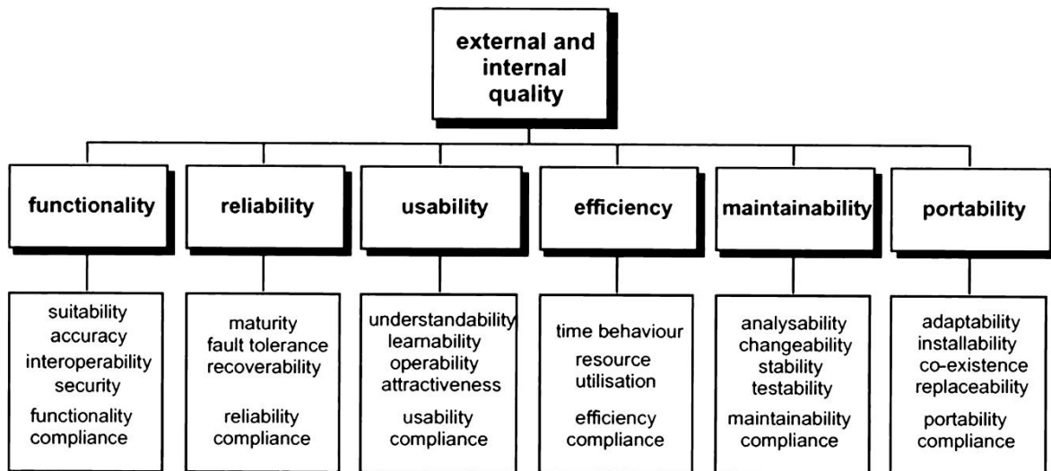
Figure 1: Attributs définis dans la norme ISO 9126 (Image tirée du cours IHDCM031 – Partie 5 – slide 33).
