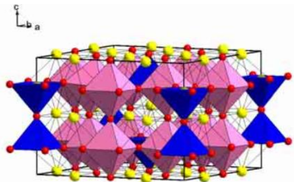
FIGURE 8 – PEROVSKITE A BASE DE STRONTIUM \text{SrFeO}_{2,875} PRESENTANT DES LACUNES D'OXYGENE, ABAISSANT AINSI LA SYMETRIE DE LA STRUCTURE (TIRE DE JOHNSON ET AL. 1 )
