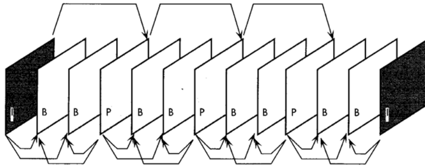
Figure 2.7 - Séquence MPEG-1 avec M=3 et N=12
