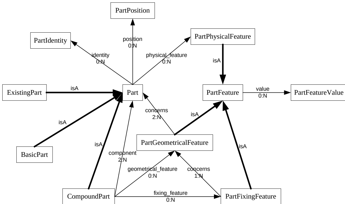
Figure 1.2 : Description graphique des classes générales du pattern Part
