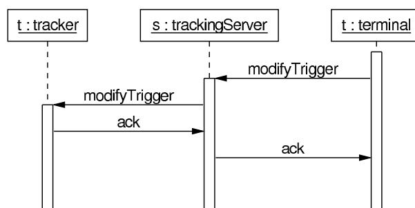
FIG. 5.4 – Modifier trigger
