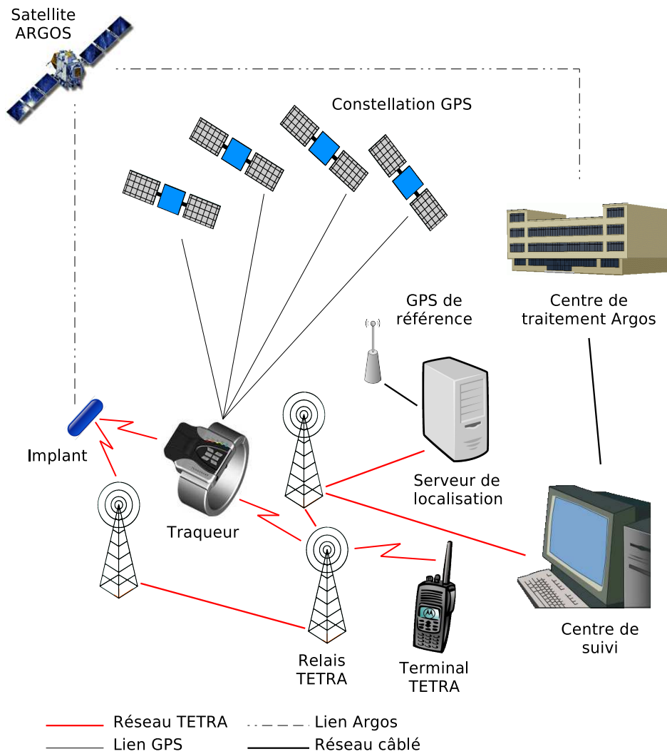
FIG. 3.2 – Architecture réseau
