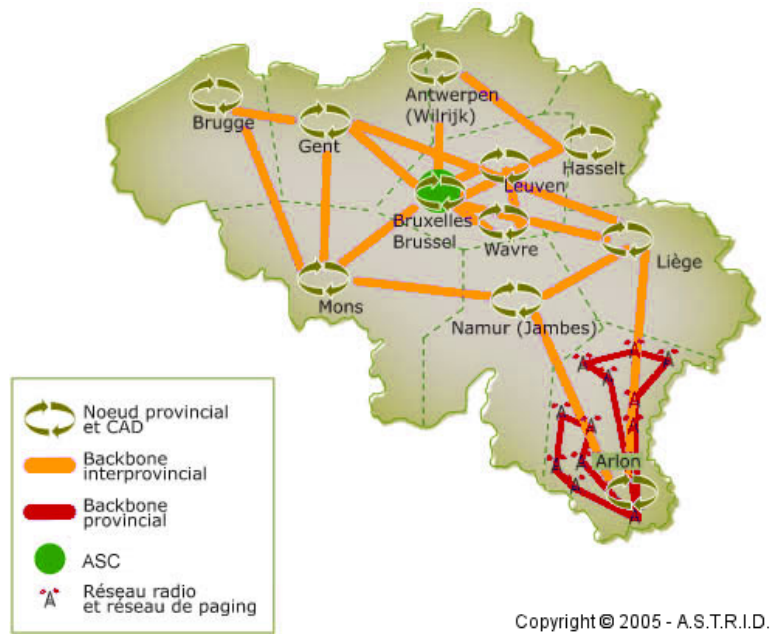
FIG. 1.1 – L'infrastructure ASTRID
