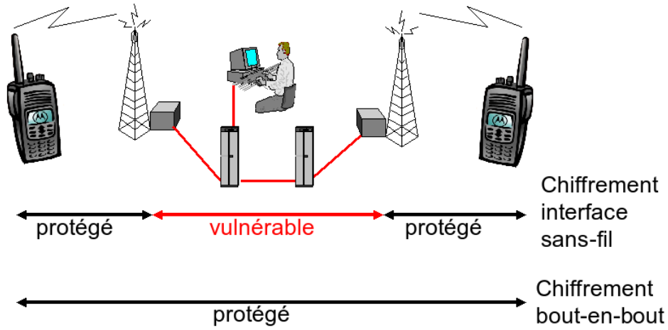
FIG. 8.3 – Sécurité TETRA
