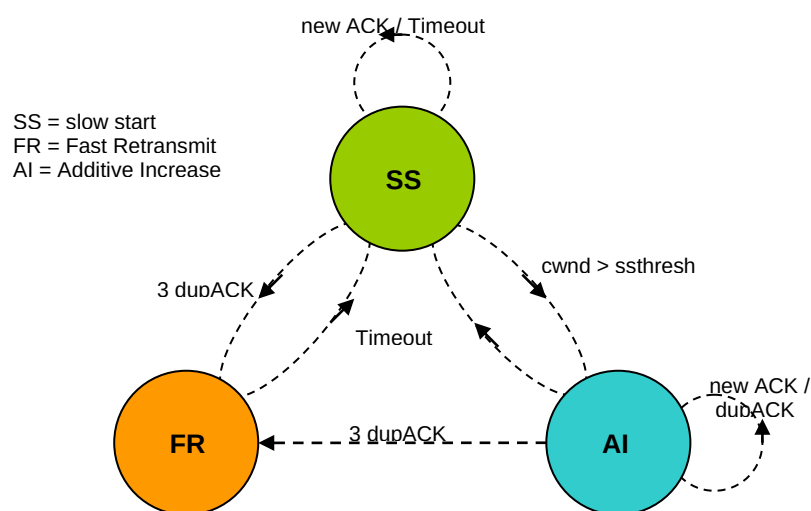
Figure 6 : états de TCP Tahoe
