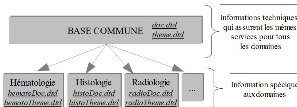
Illustration 33: Extension de la base commune du modèle de contenu, avec indication des dtd 's (sans scénarios)
