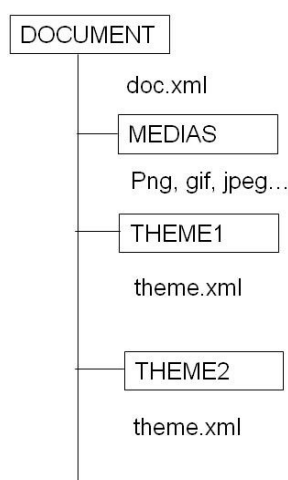
Illustration 31: Présentation de l'arborescence du « package » représentant un contenu (sans scénarios)
