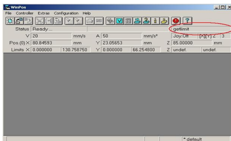
Illustration 14: L'interface de WinPos et l'affichage des commandes envoyées
