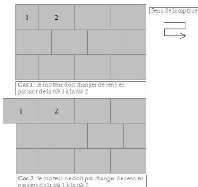
Illustration 27: Illustration de la structure d'une méga-image après coregistration
