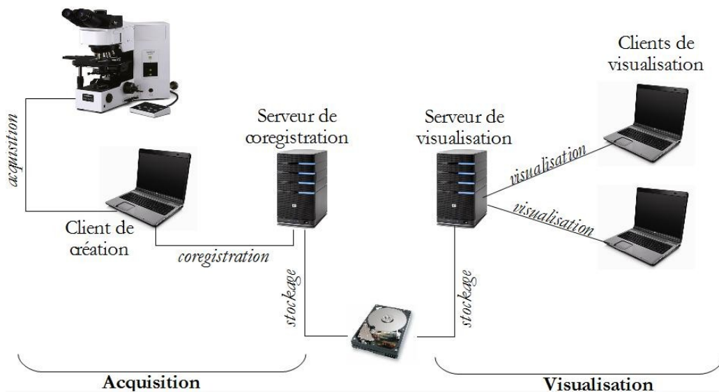
Illustration 7: Architecture générale du microscope virtuel
