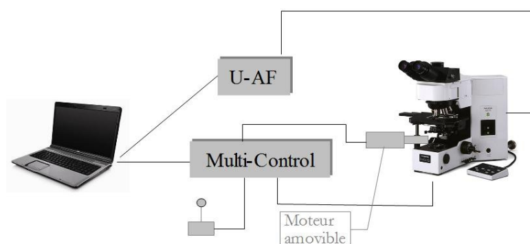
Illustration 29: Schéma simplifié du branchement entre l'ordinateur de contrôle, l' U-AF , le Multi-Control , le joystick et le microscope
