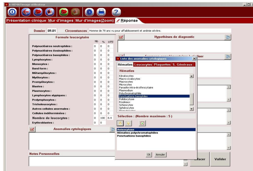
Illustration 4: GUI de l'application e-hematimage (sélection d'une réponse)
