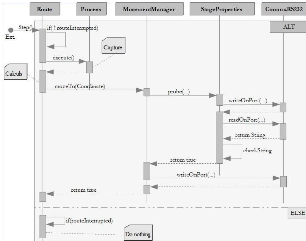
Illustration 26: Diagramme de séquence de l'exécution d'une étape dans une route prédéfinie
