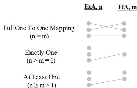
Illustration 42: Schéma des correspondances possibles entre les réponses attendues et les réponses effectives
