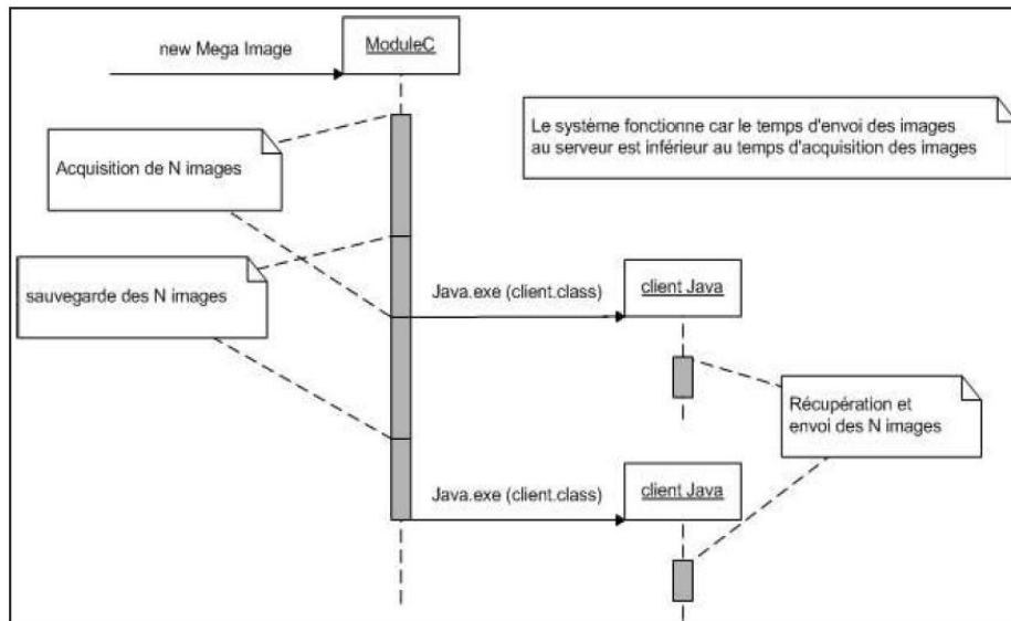
Illustration 47: Communication entre le module C et le client Java (tiré de [zuy03])
