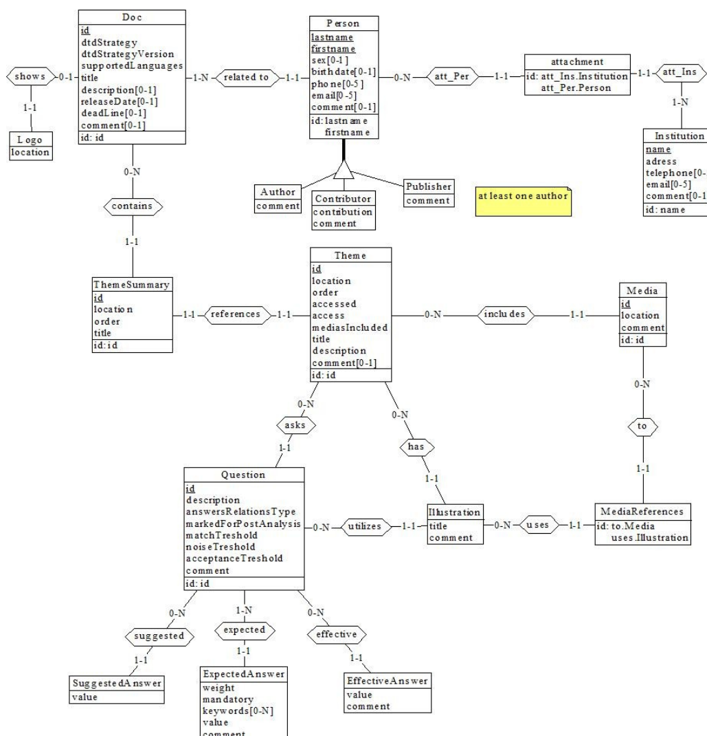
Illustration 35: Schéma ERA de la stratégie DTD pour l'hématologie (ou stratégie générale) (sans les scénarios)
