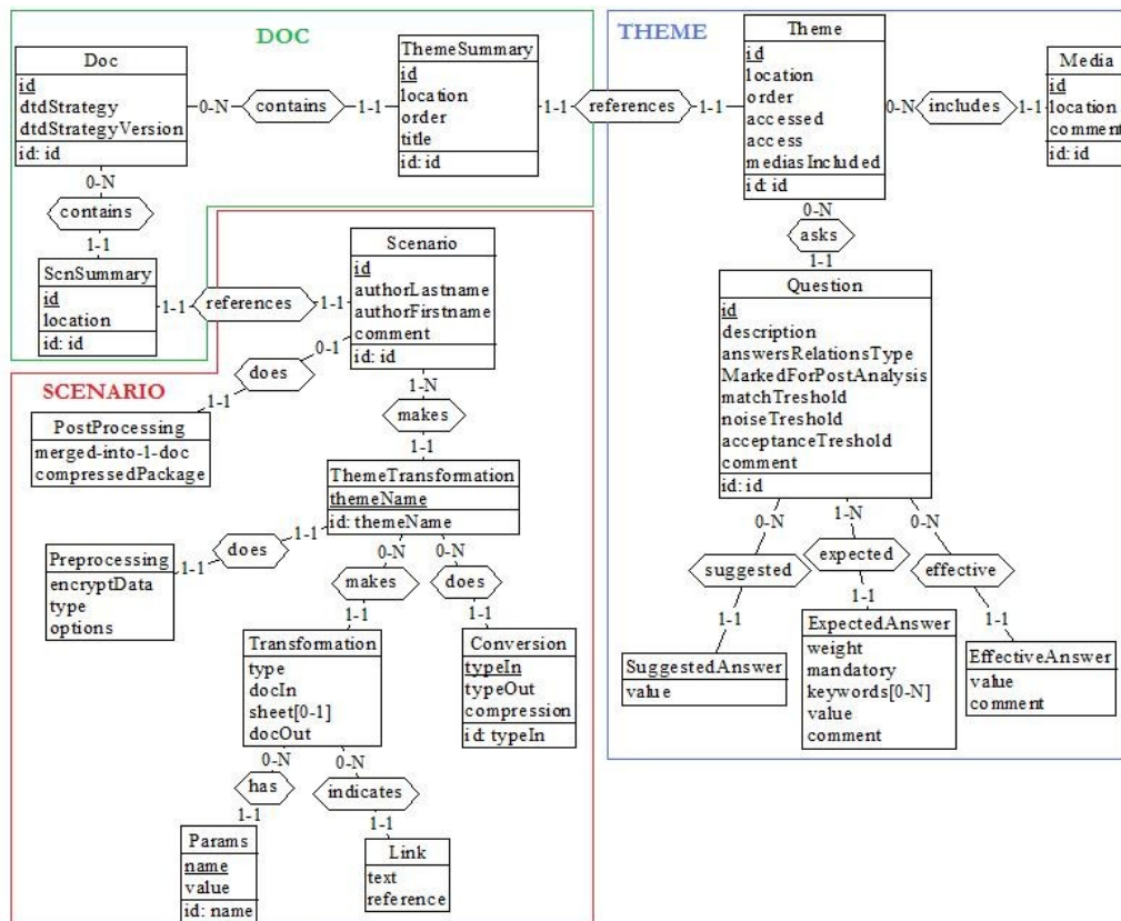
Illustration 38: Schéma ERA de la base commune du modèle de contenu
