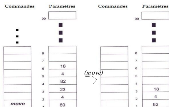
Illustration 13: Effet de l'application d'une commande "move" sur les stacks
