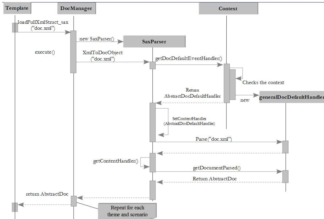
Illustration 48: Diagramme de séquence du parsing d'un document xml depuis un template
