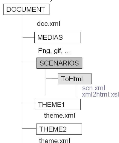
Illustration 36: Présentation de l'arborescence du « package » représentant un contenu avec les scénarios
