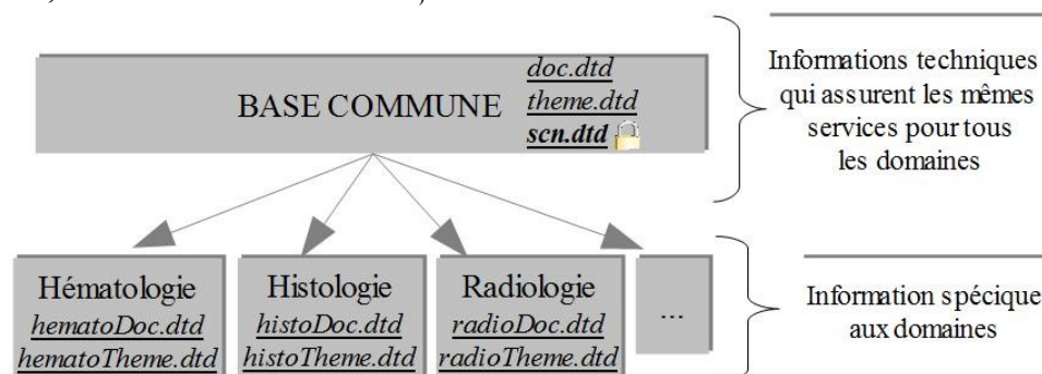
Illustration 37: Extension de la base commune du modèle de contenu avec les scénarios (qui sont non extensibles)
