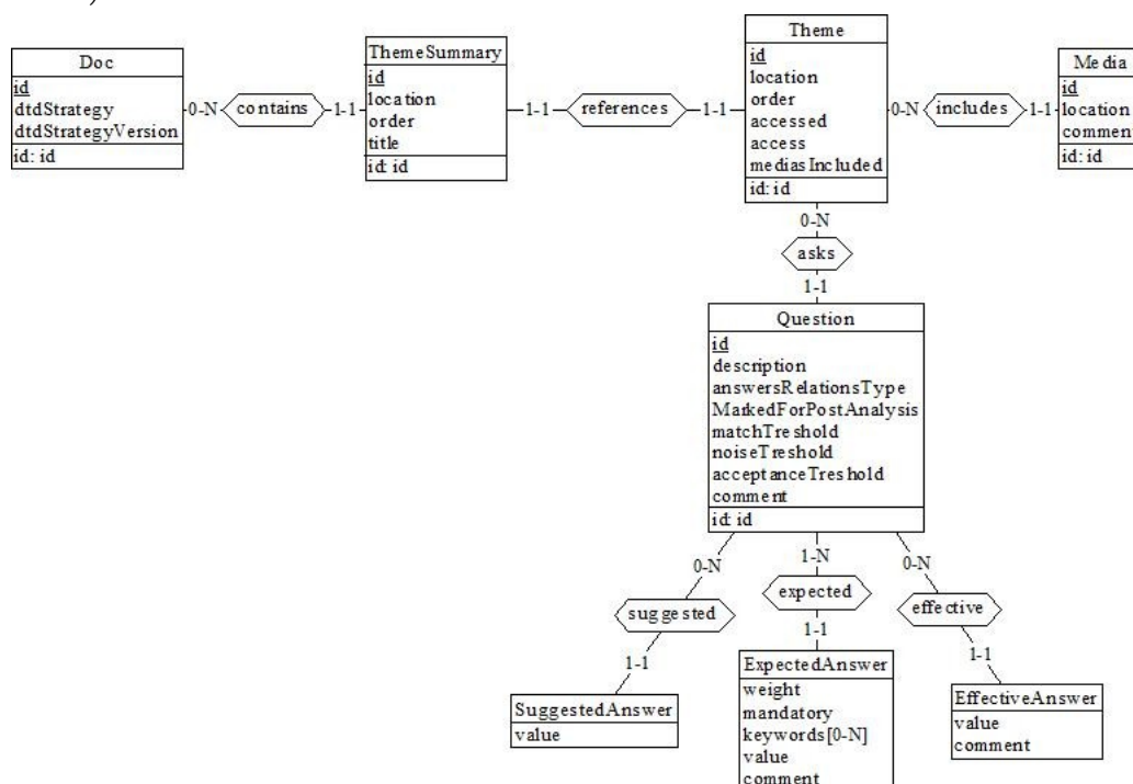
Illustration 34: Schéma ERA de la base commune du modèle de contenu (sans scénarios)
