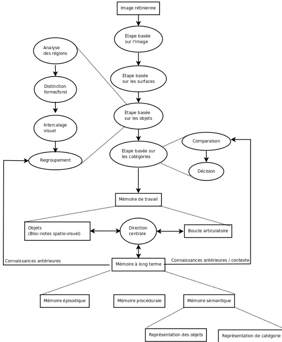
FIG. 2.1: Théorie de la compréhension logicielle par la vision (adaptée de [Gué05]). Les boîtes représentent les représentations d'une image, les cercles sont les processus, les flèches décrivent le flux d'information, les lignes pointillées montrent les décompositions. L'absence de représentation entre les processus n'en exclut pas l'existence mais simplifie le flux.
