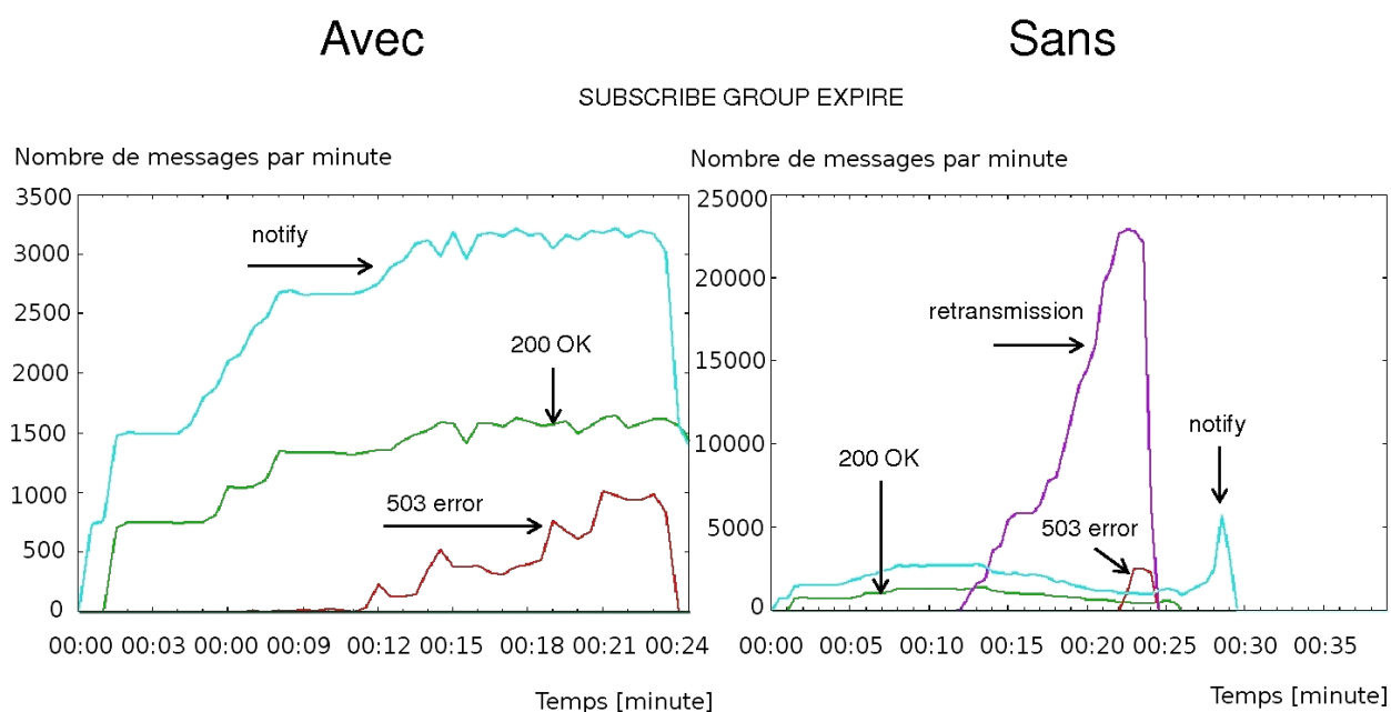
Figure 6.11 – L'injection des messages SUBSCRIBE GROUP à taux variable
