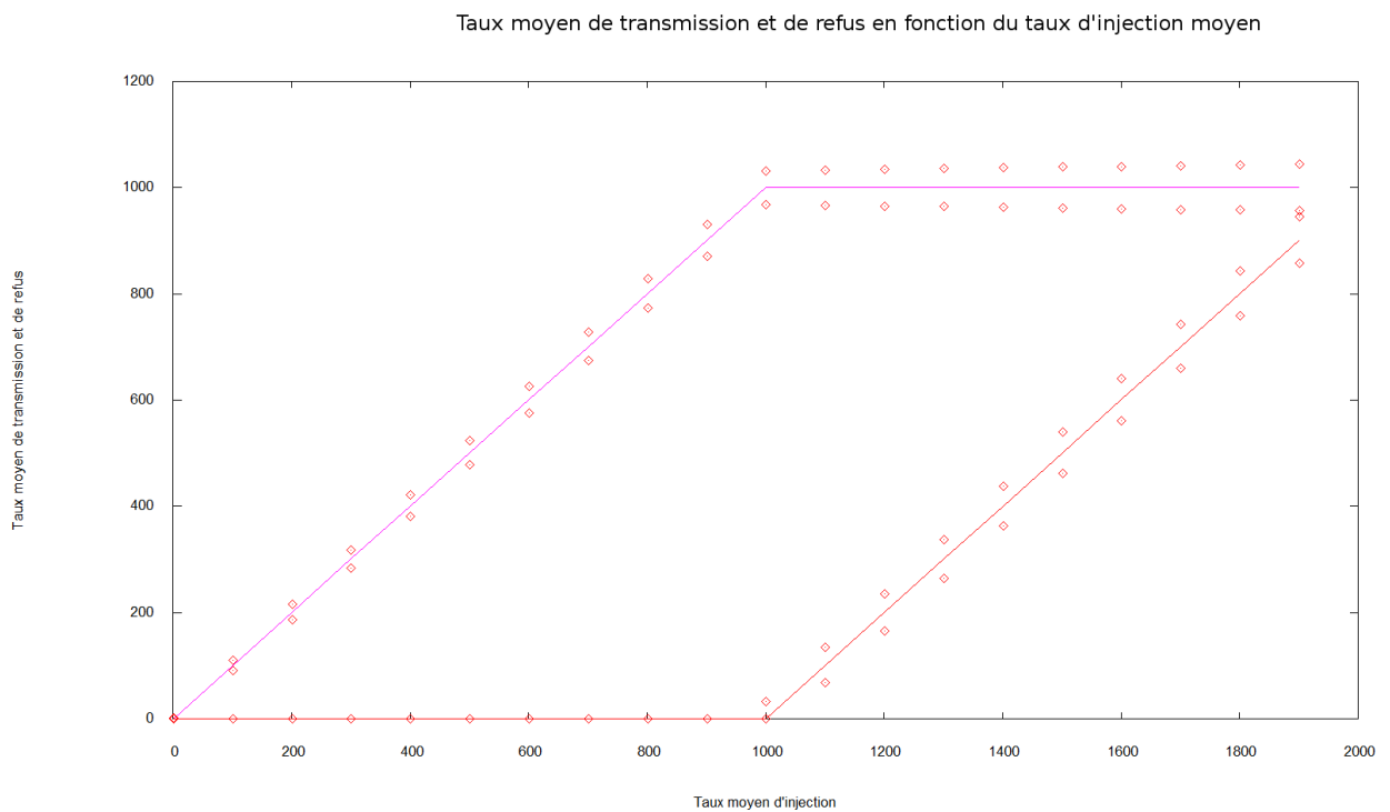
Figure 5.10 – Evolution des taux moyens de transmission et de refus en fonction du taux moyen de messages injectés. Les lignes en pointillé montrent l'écart-type autour des lignes pleines qui représentent des valeurs moyennes.
