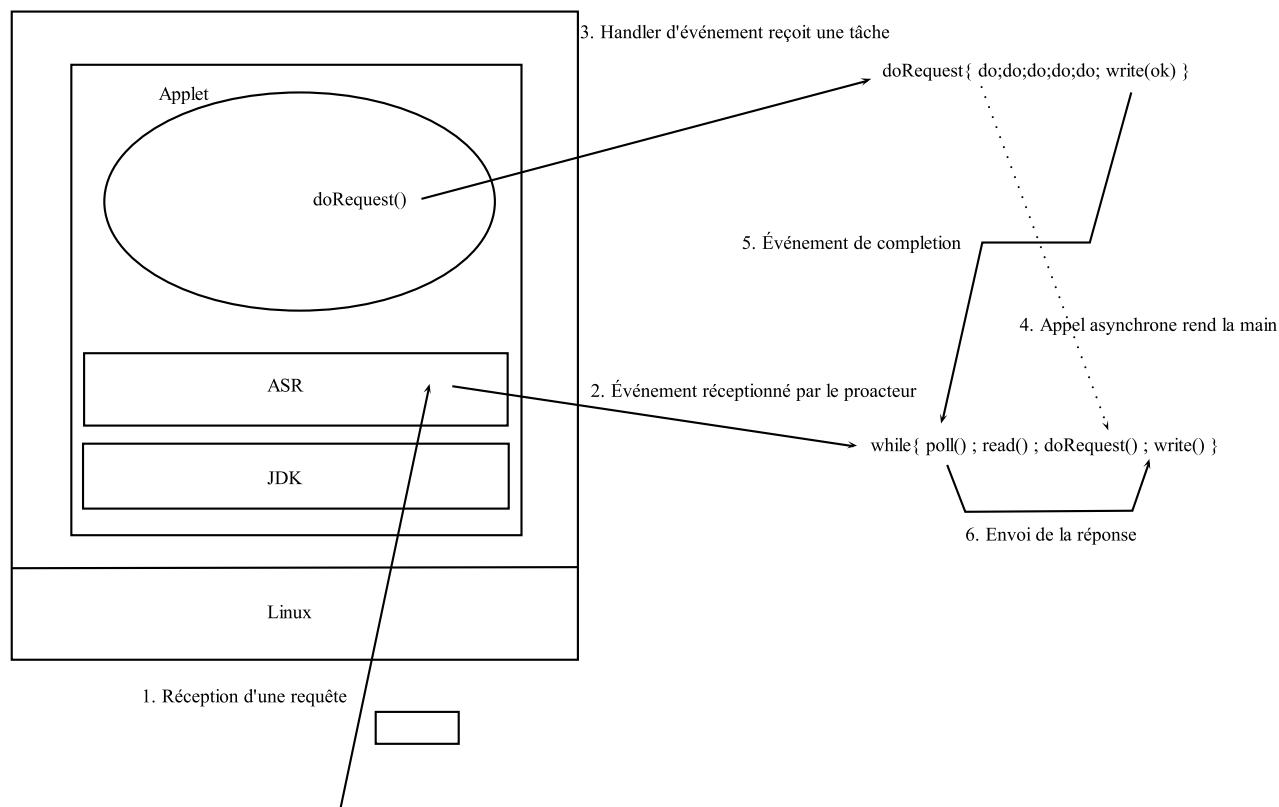
Figure 2.5 – Le pattern Proactor est implémenté dans l'ASR.
