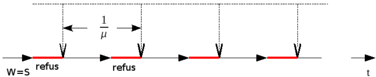
Figure 5.4 – L'agent n'est pas surchargé, car un nombre suffisant de messages est refusé.
