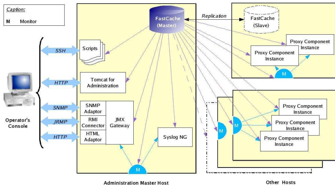
Figure 2.7 – Le schéma global de l'administration de l'ASR.
