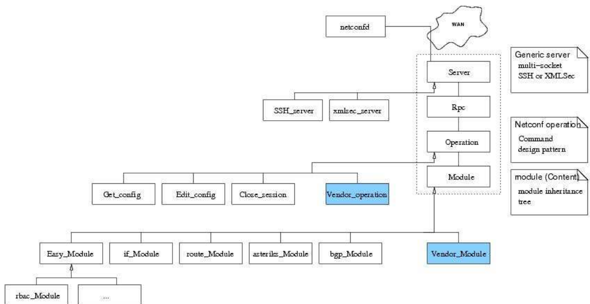
Figure 25: L'architecture multi-couches de l'agent YencaP [12,26]
