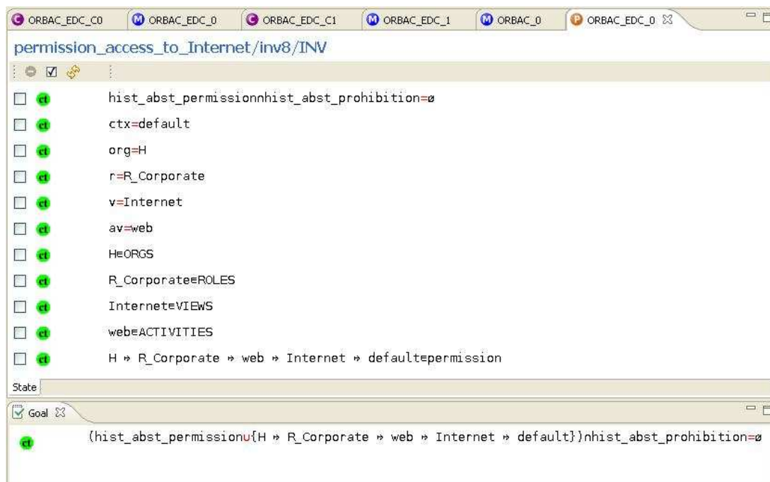
Figure 32 : Obligation de preuve générée sur l'invariant inv8
