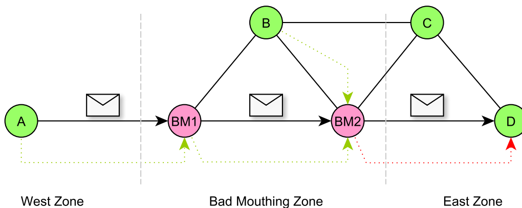
FIGURE 2.8: Comportement malicieux de type Bad-Mouthing en environnement sans fil
