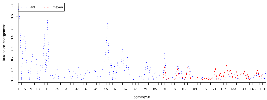
FIGURE 5.5 – Taux de co-changement de LinuxTools
