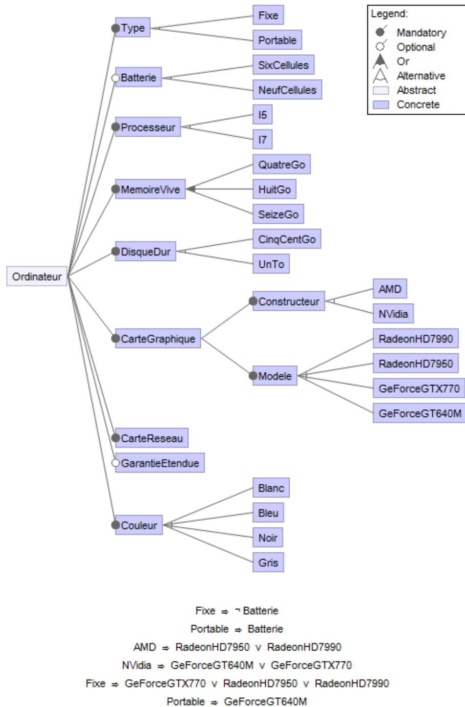
FIGURE 4.2 – Feature Model - Ligne d'ordinateurs
