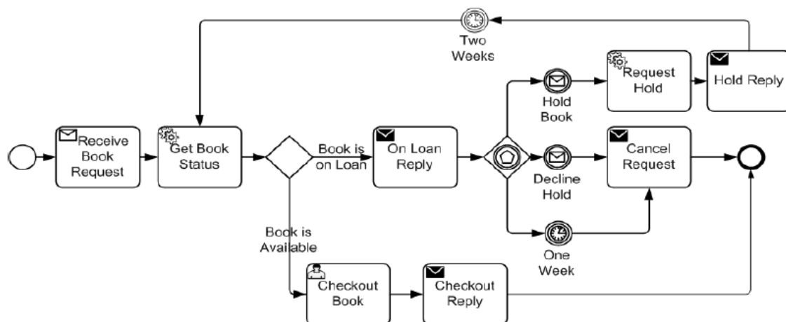
FIGURE 3.1 – BPMN 2.0 : Exemple
