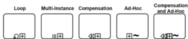
FIGURE 3.3 – BPMN 2.0 : Types de sous-processus
