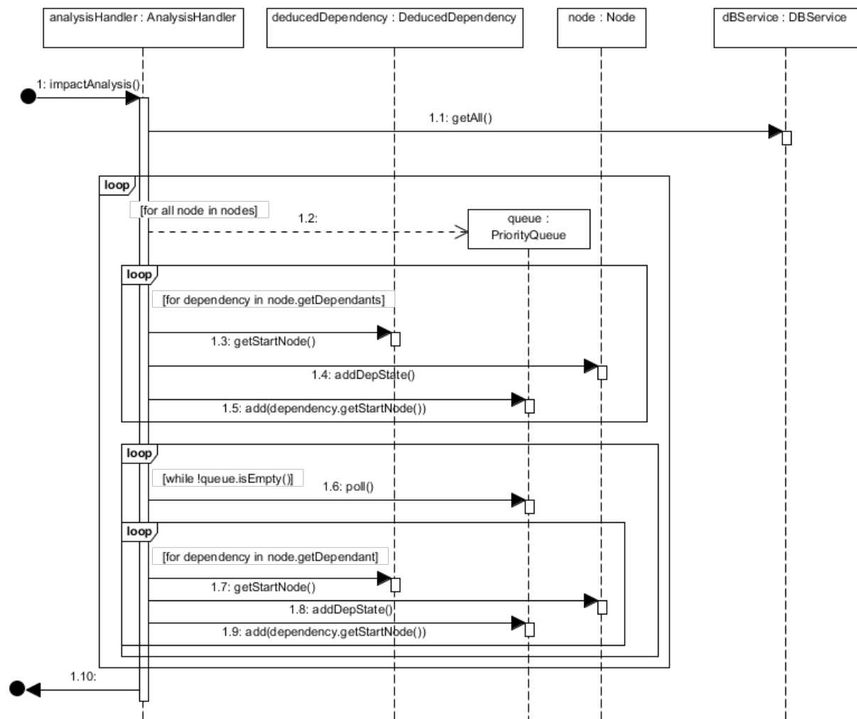
FIGURE 8.7 – Diagramme de séquence - Analyse d'impact
