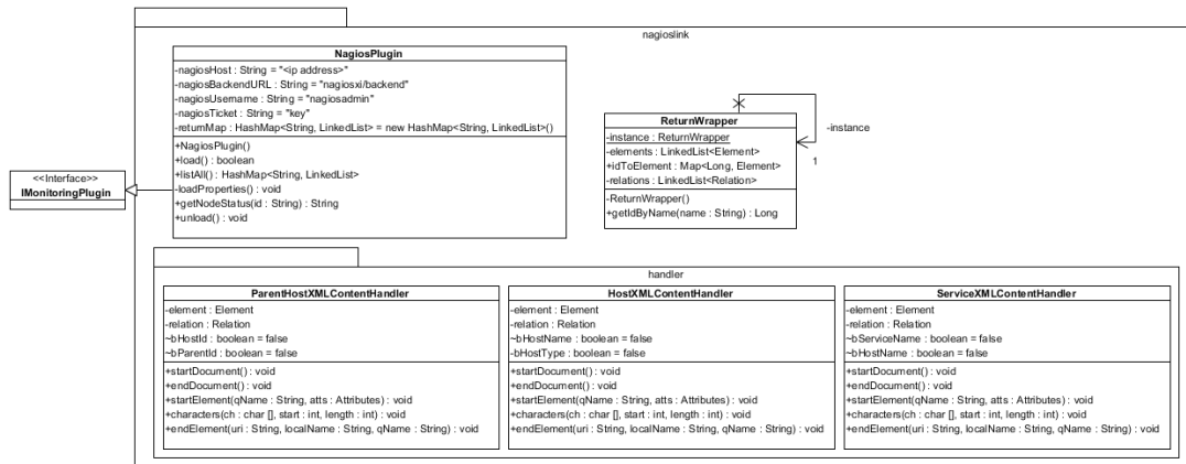
FIGURE 8.8 – Diagramme de classe - Plugin de connexion Nagios
