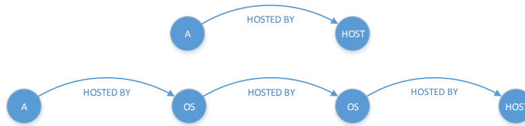
FIGURE 5.2 – Relation d'hébergement
