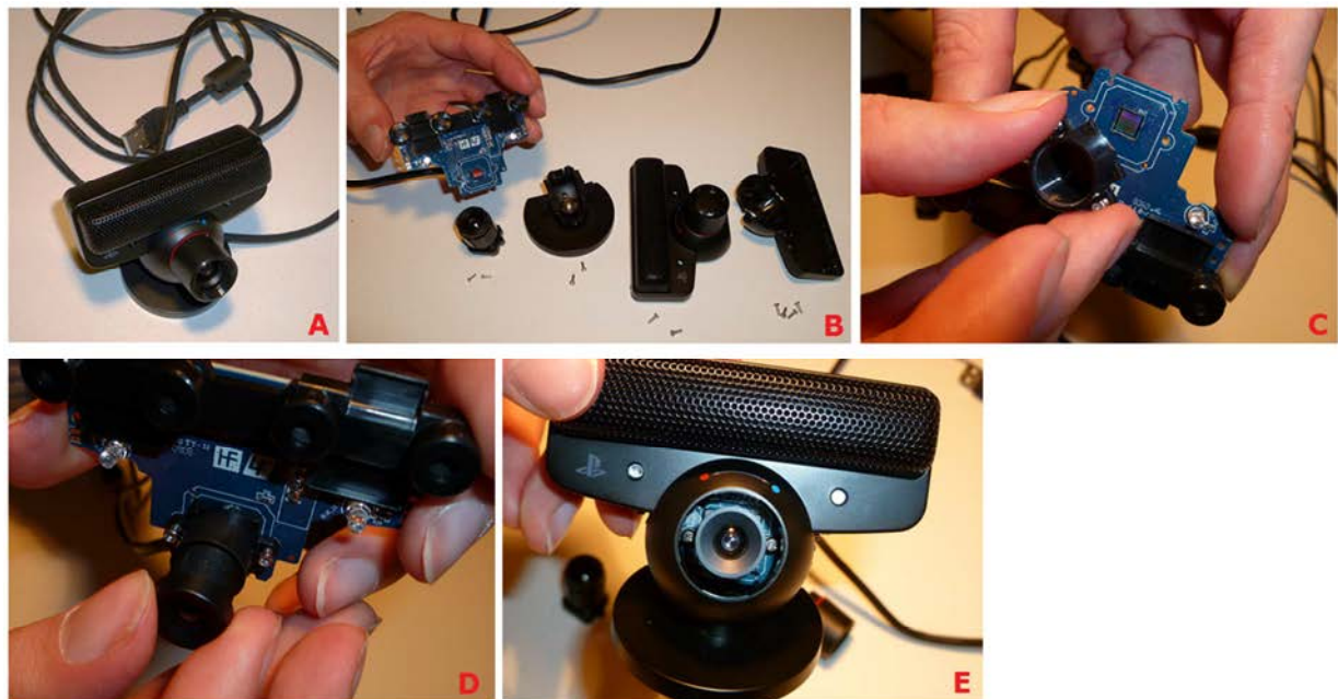
Figure 6.7 : Les étapes réalisées pour changer l'objectif de la PS3Eye : (A) PS3Eye originale ; (B) Démontage complet de la PS3Eye ; (C) Montage de la nouvelle fixation objectif ; (D) Vissage du nouvel objectif ; (E) PS3Eye remontée avec le nouvel objectif.
