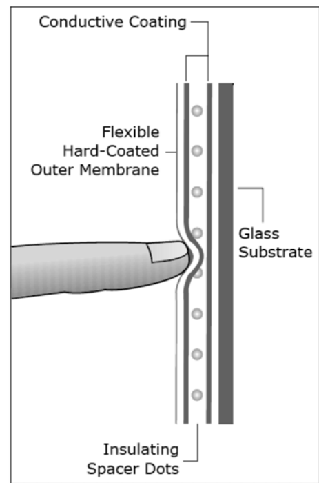
Figure 2.6 : Schéma de la technologie résistive. Source : [Schöning, et al., 2008, p. 3]
