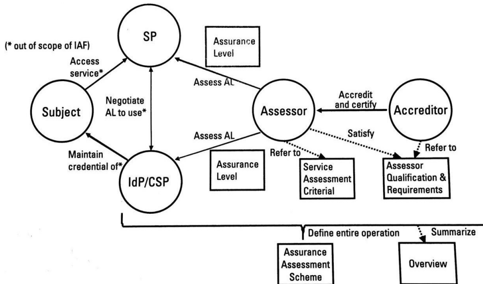
FIGURE 1.6 – Une vue d'ensemble de l'IAF [7]
