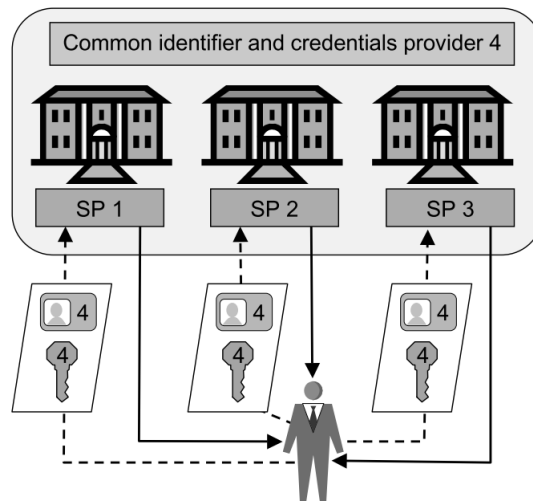
FIGURE 1.10 – Gestion de l'identité centralisée : identité commune [20]
