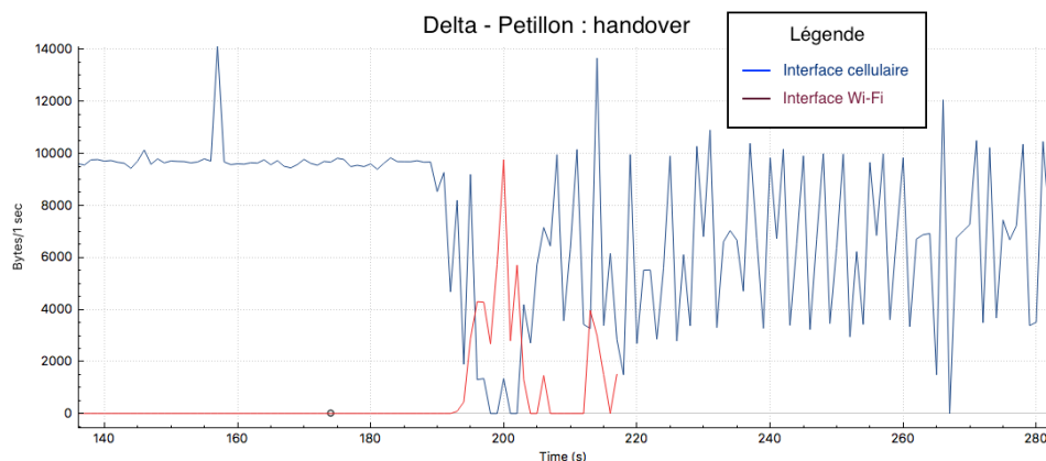
FIGURE 5.2 – Streaming audio dans le métro - handover
