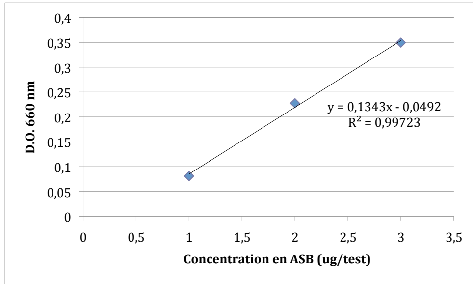
Figure 2.2. Exemple d'une droite d'étalonnage à l'ASB :
