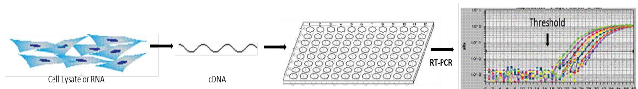
Figure 2.5: Principe de la RT-PCR en temps réel.
