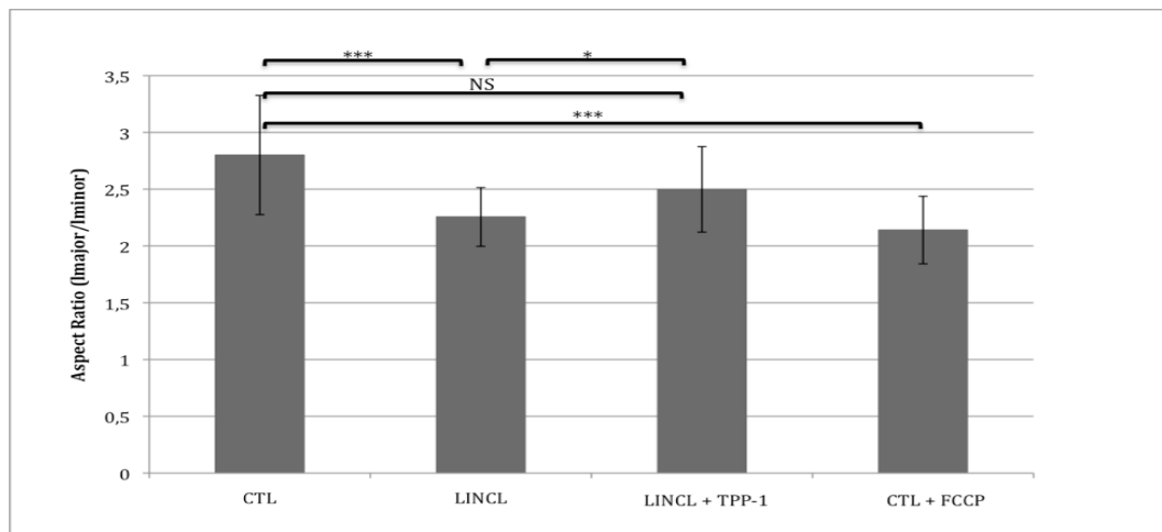
Figure 3.4 : Quantification de la fragmentation du réseau mitochondrial (Aspect Ratio)
