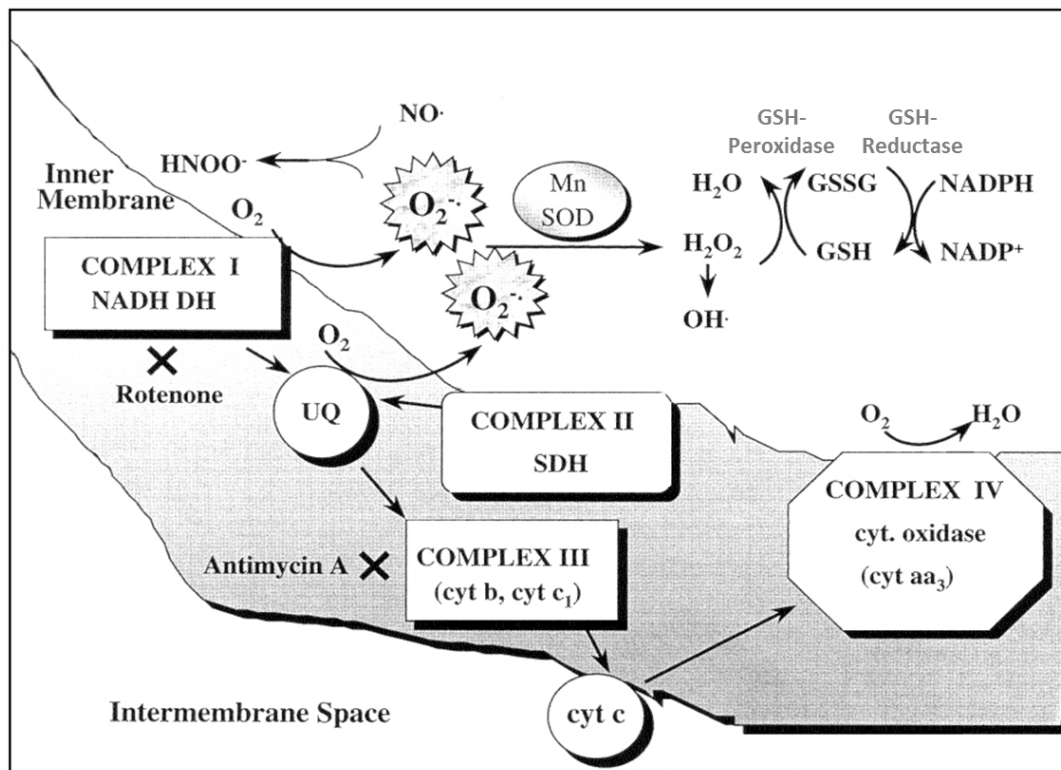
Figure 1.16. Production et détoxification des ROS par le Glutathion
