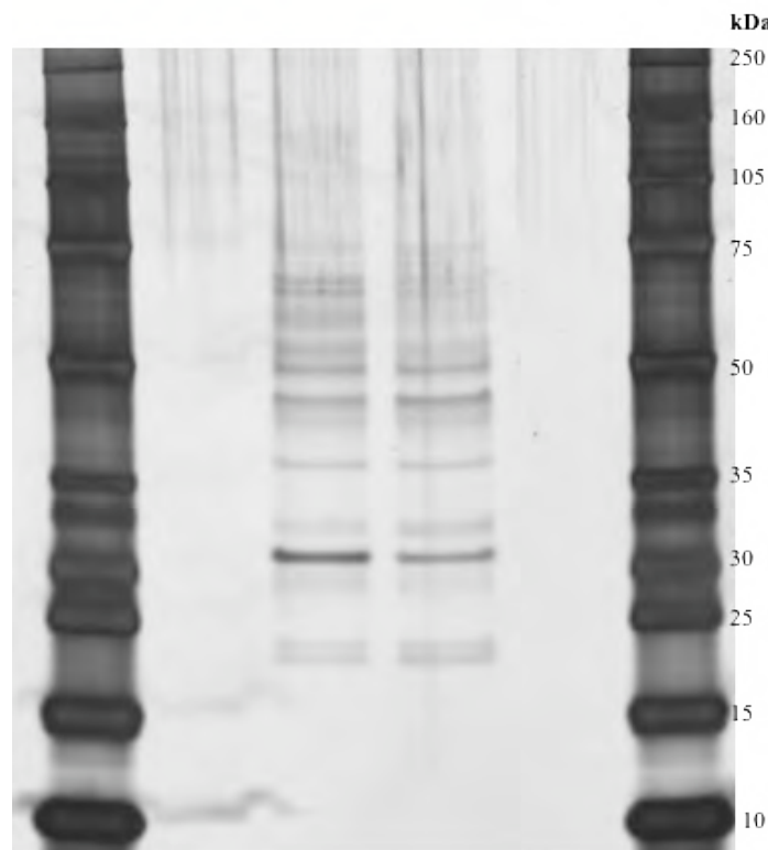
Figure 18. Purification TAP de Plh1. Les fractions d'éluion ont été séparées par SDS-PAGE et le gel a été coloré à l'argent.
