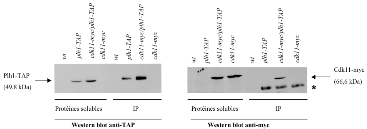
Figure 14. Coimmunoprécipitation Plh1-TAP/Cdk11-myc . Les protéines solubles et les protéines immunoprécipitées (anti TAP) et les protéines solubles des souches wt, plh1-TAP , cdk11-myc et plh1-TAP/cdk11-myc ont été séparées par SDS-PAGE. Un Western Blot utilisant l'anticorps PAP et un Western Blot utilisant l'anticorps anti-myc ont été réalisés.
