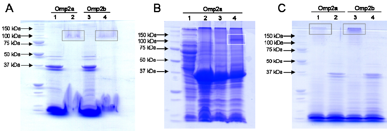
Figure 17. Gels SDS-PAGE des protéines renaturées au zwittergent 3-14 à A) 10%, B) 1% et C) 0,14%. Les tailles attendues pour les formes dénaturées sont d'environ 39,42 kDa et de 40,38 kDa respectivement pour Omp2a et Omp2b. En ce qui concerne les formes renaturées sous forme trimérique, les tailles attendues pour Omp2a et Omp2b sont d'environ 118,23 kDa et 121,14 kDa respectivement. (A) Ce premier gel montre les profils de migration des Omp2a et Omp2b dénaturées dans les puits 1 et 3 respectivement et de ces mêmes porines renaturées par dilution 1:1 dans du zwittergent 3-14 à 10% (dissout dans le tampon TEN) dans les puits 2 et 4 respectivement. (B) Ce second gel ne concerne que la renaturation d'Omp2a avec du zwittergent 3-14 à 1%. Dans le puits 1 a migré la fraction soluble obtenue lors de la lyse bactérienne. Le puits 2 présente le profil de migration des corps d'inclusion solubilisés. Enfin, respectivement dans les puits 3 et 4 ont migré Omp2a renaturée sans ou avec l'étape de sonication (cfr Matériels et méthodes). (C) Dans les puits 2 et 4 ont migrés les corps d'inclusion solubilisés contenant Omp2a et Omp2b. La migration de ces mêmes OMPs renaturées avec du zwittergent 3-14 de concentration 0,14% est visualisable dans les puits 1, pour Omp2a, et 3, pour Omp2b.
