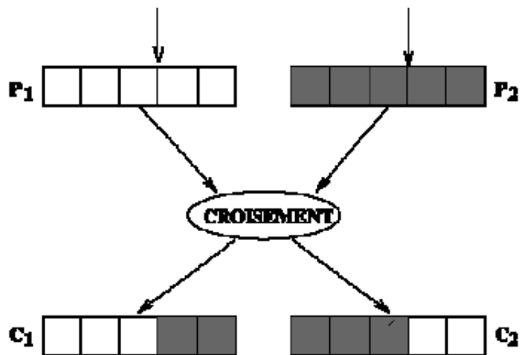
Figure 3.3: Croisement avec un seul point de croisement
