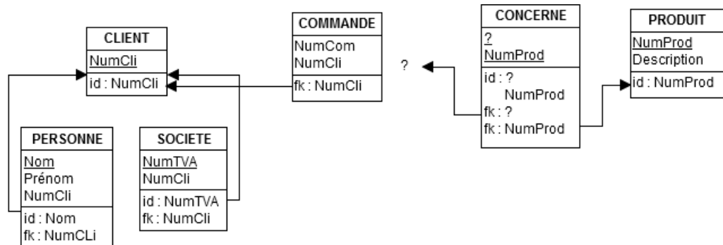
Figure 4.12: Exemple équivalent en schéma relationnel
