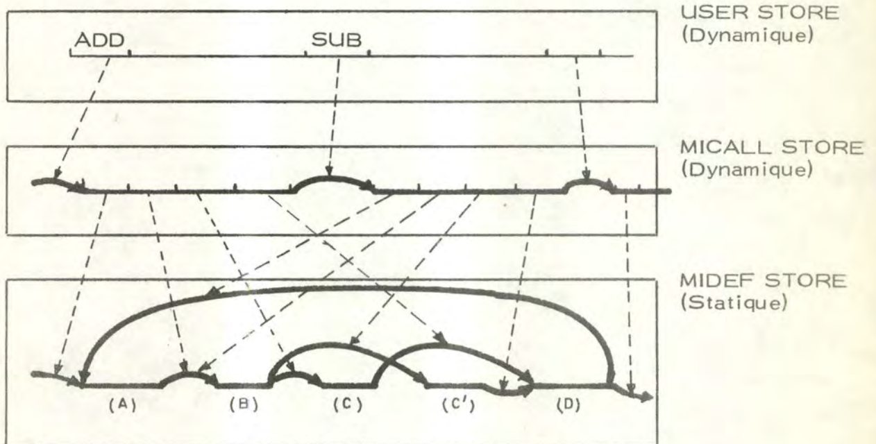
Fig. 1-2 : Interpréteur micro-programmé à deux étapes d'interprétation. (V. légende)
