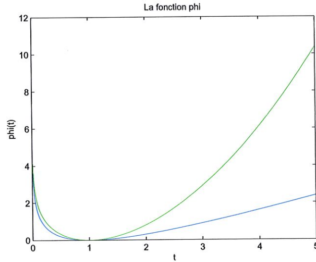
FIG. 3.1 – Fonction \varphi
