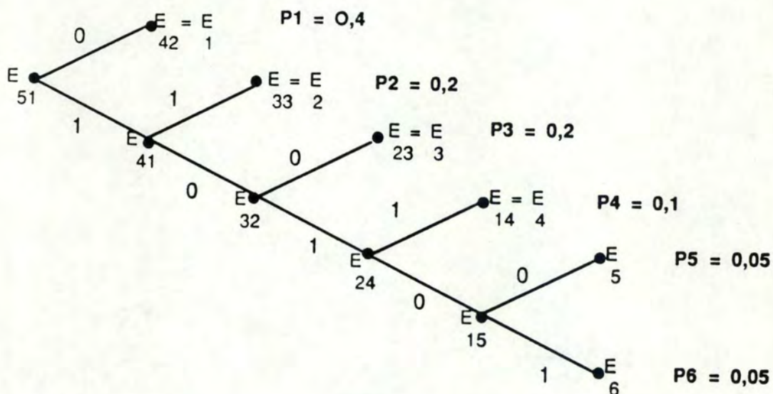
fig.2.6 Attribution des mots de code.
