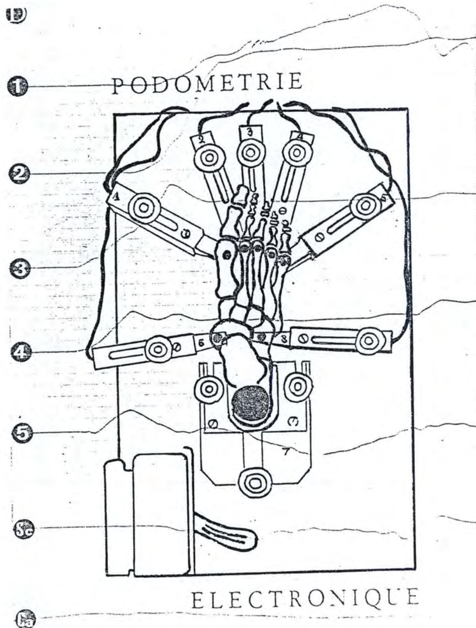
fig. 12. : Schéma du podomètre électronique illustrant la position respective des palpeurs et des points explorés
