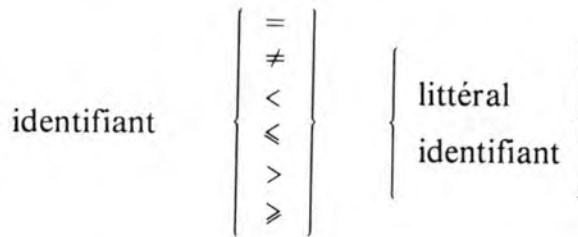
fig. 5.1.7. – format des conditions élémentaires
