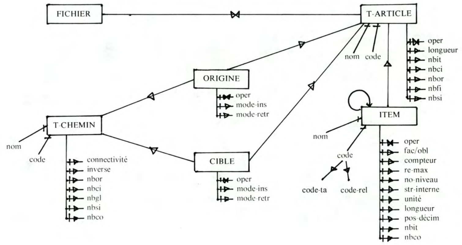
Schéma conceptuel de la BD-schéma (suite).
