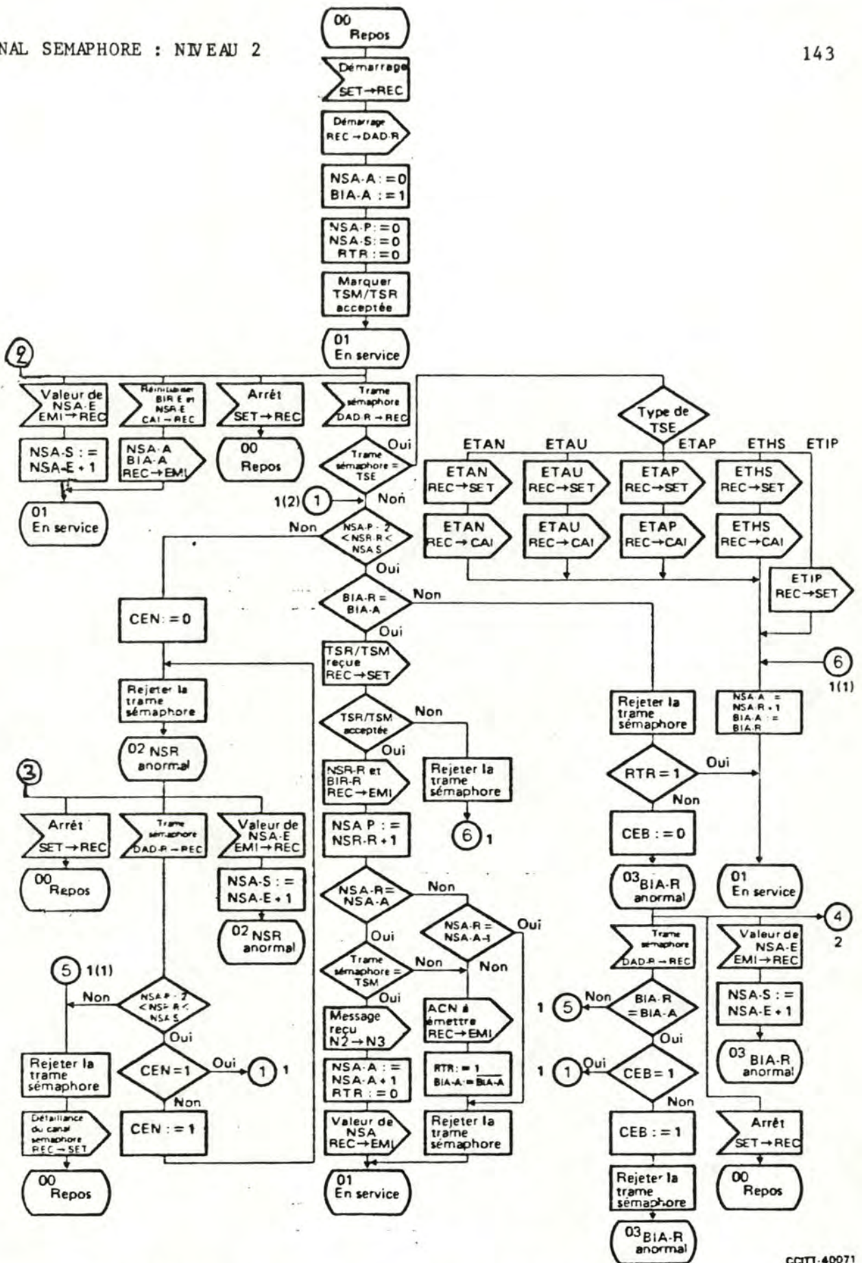
Figure VI 4 6: commande de la réception (méthode de base)
