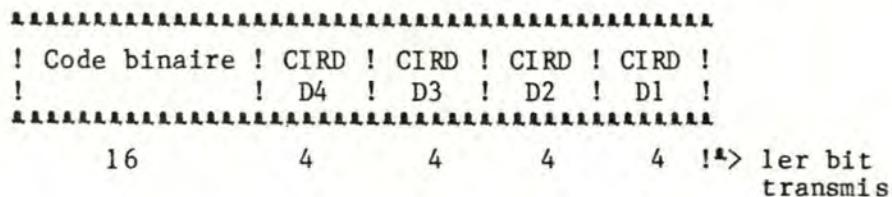
Figure II A 6: Format du code de verrouillage
