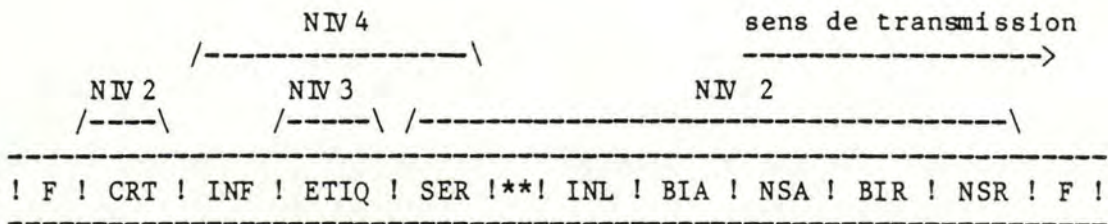
Figure 3 A 5: Trame sémaphore de message
