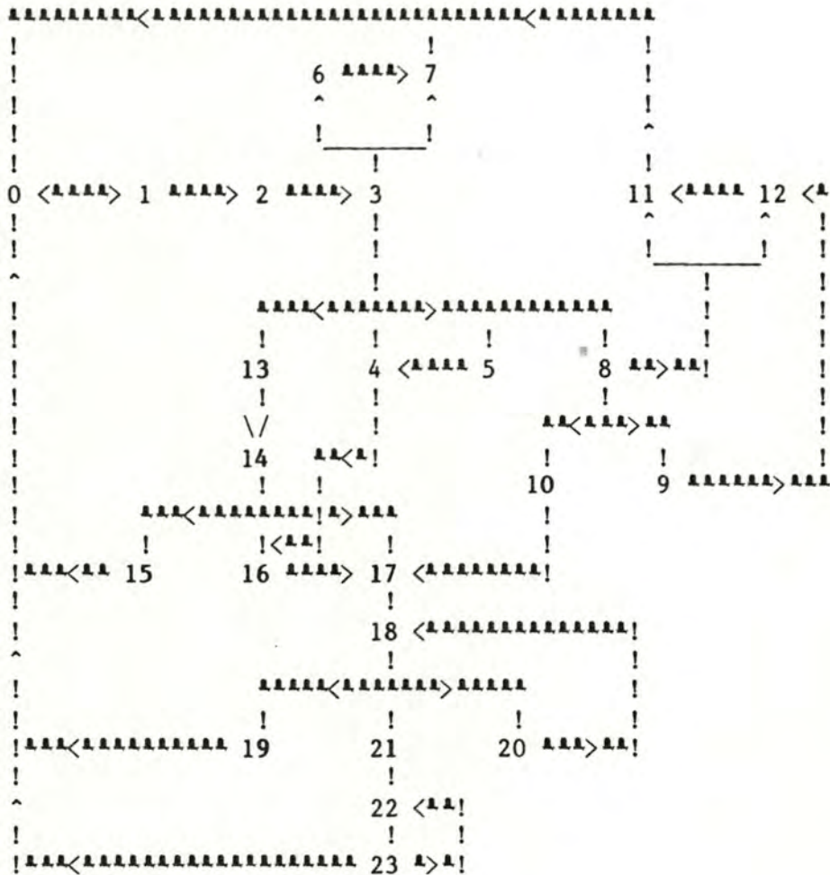
Figure VII A 5: Graphe associé à la table de décision côté appelant
