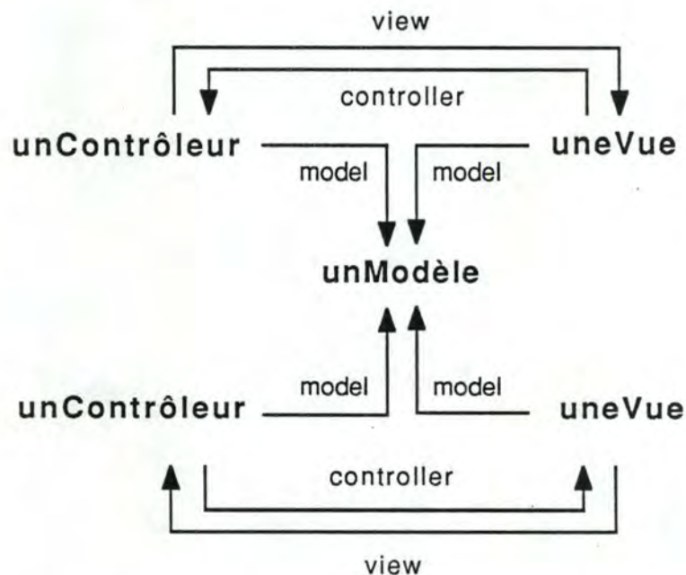
figure 4.7: Schématisation des relations entre un modèle, ses deux vues et ses deux contrôleurs
