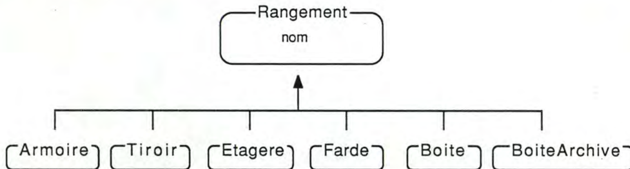
figure 6.4: Hiérarchie des objets de rangement et leur variable d'instance
