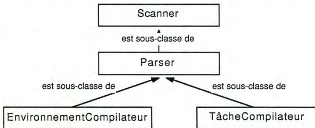
figure 9.2: Les classes EnvironnementCompilateur, TâcheCompilateur et leurs super-classes
