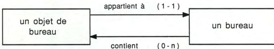
figure 6.11: L'association d'appartenance
