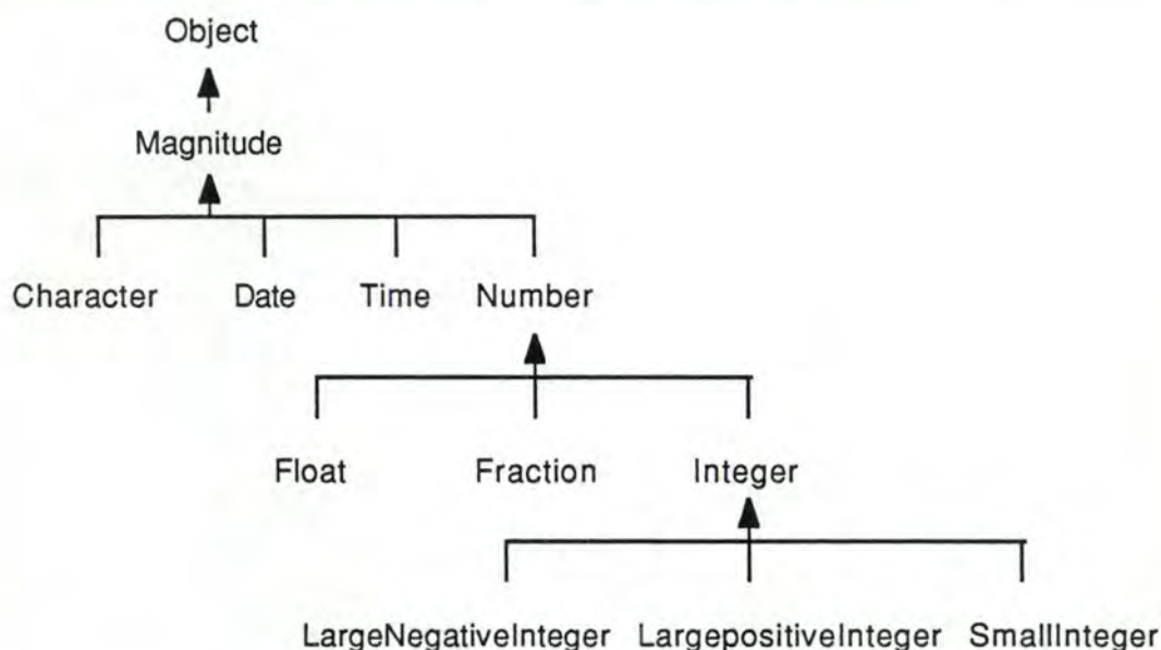
figure 4.2: La classe Number et ses sous-classes
