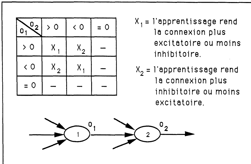
Figure IV.9. : Règle de Hebb.
