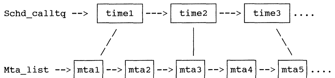
Figure 8.11: Exemple de configuration de la liste Schd_calltq.
