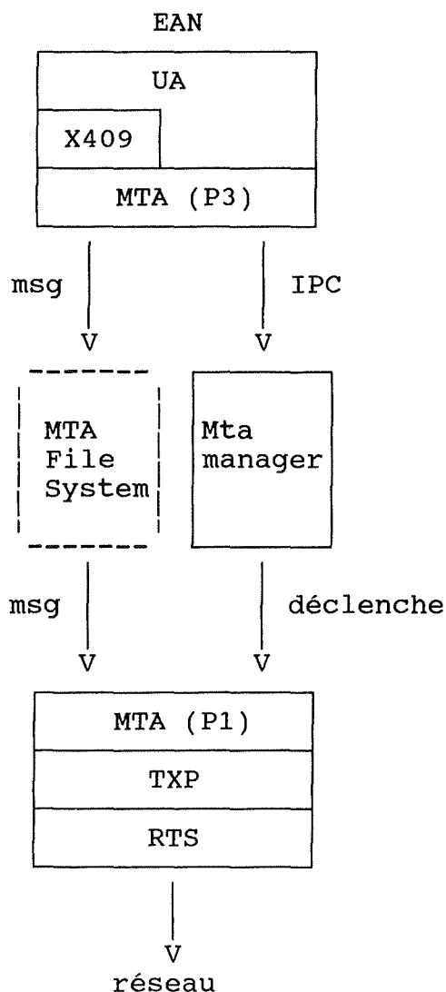
Figure 8.1: Parcours d'un message dans EAN.
