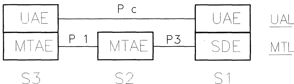
Figure 1.5 : entités et protocoles du modèle MHS
