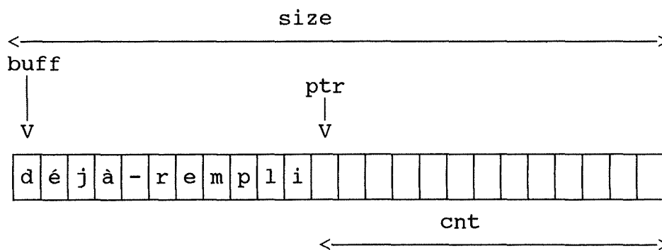
Figure 7.5: Configuration d'un IO_DESC utilisé en sortie.
