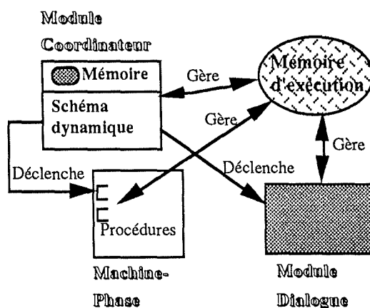
Figure VI.2 Mémoire d'exécution globale
