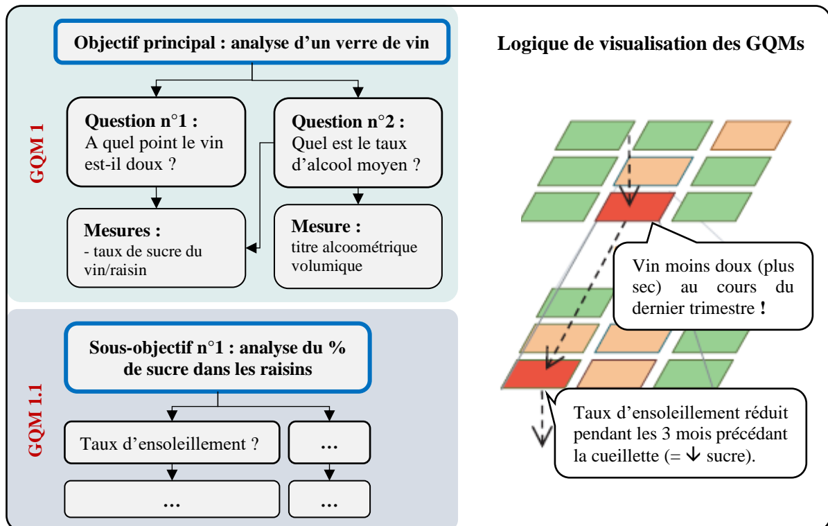
Figure 1.2 : élaboration d'un modèle GQM
