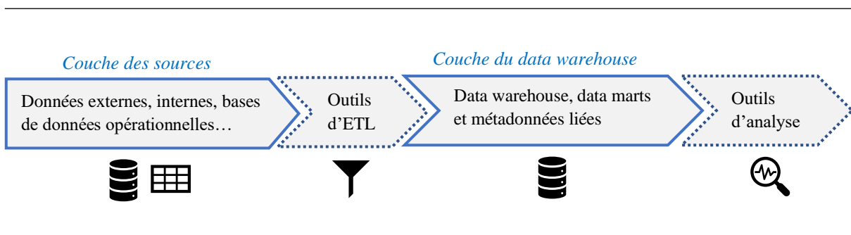
Figure 1.1 : l'architecture double couche (architecture choisie)
