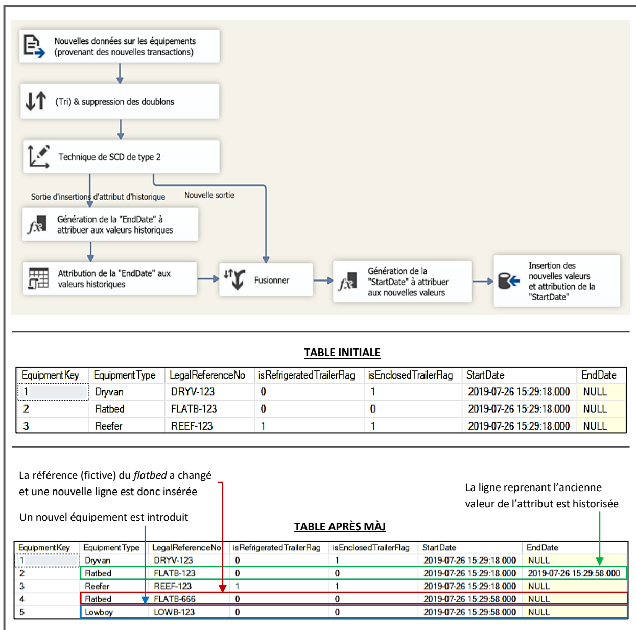
Figure 4.3 : illustration du fonctionnement des SCD de type 2
