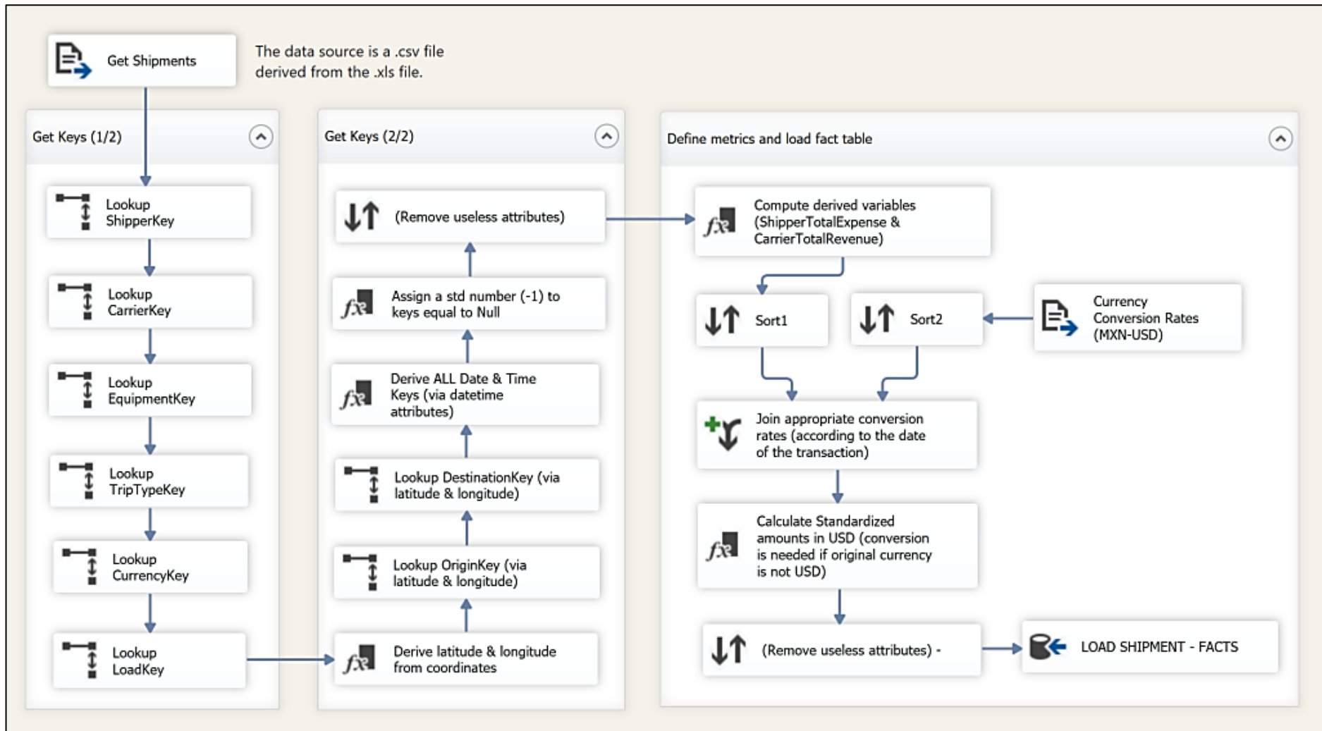
Figure A-3.3 : tâche de flux de chargement de la table de faits
