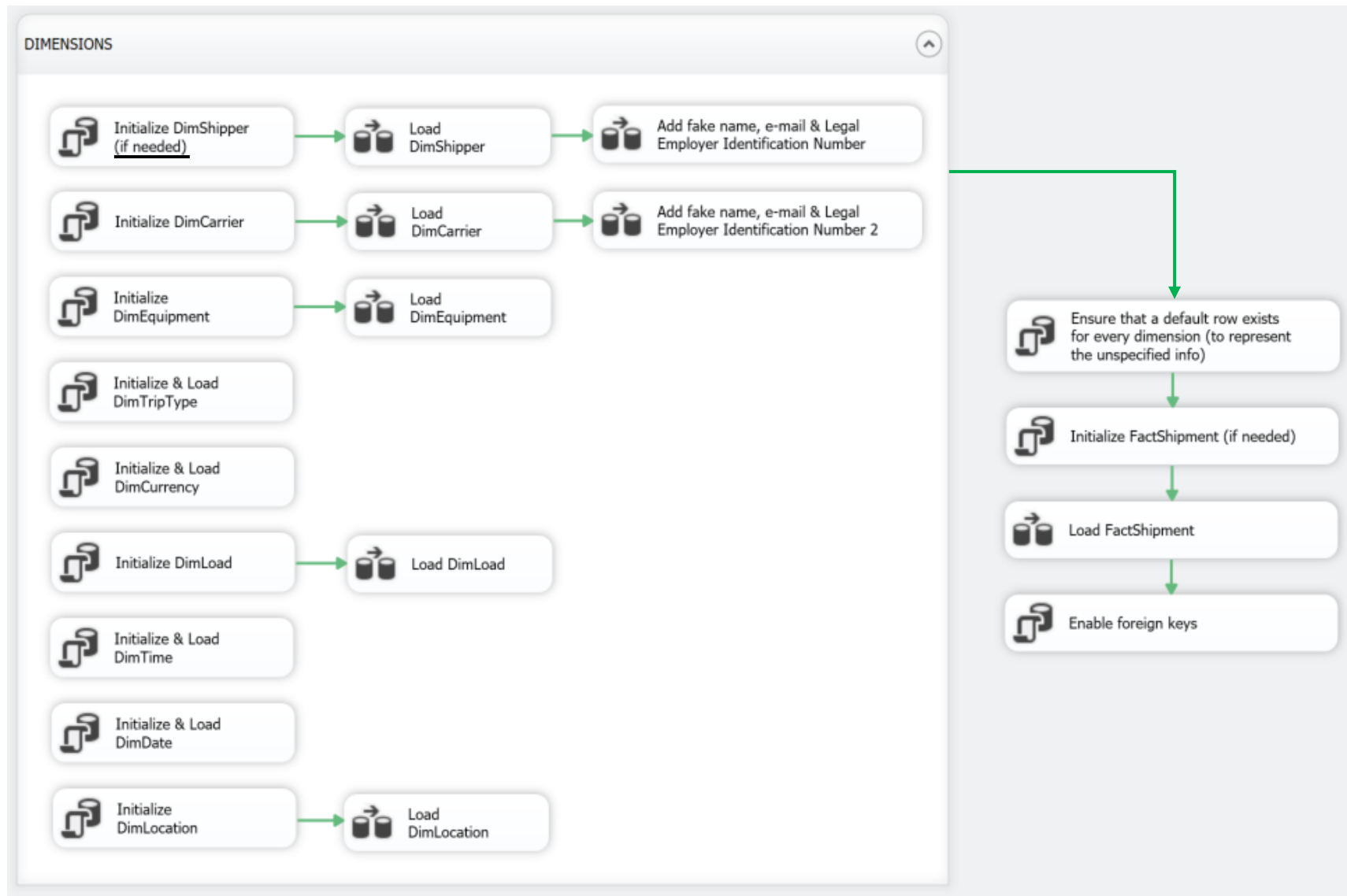
Figure 4.2 : mise en œuvre de l'ETL avec SSIS
