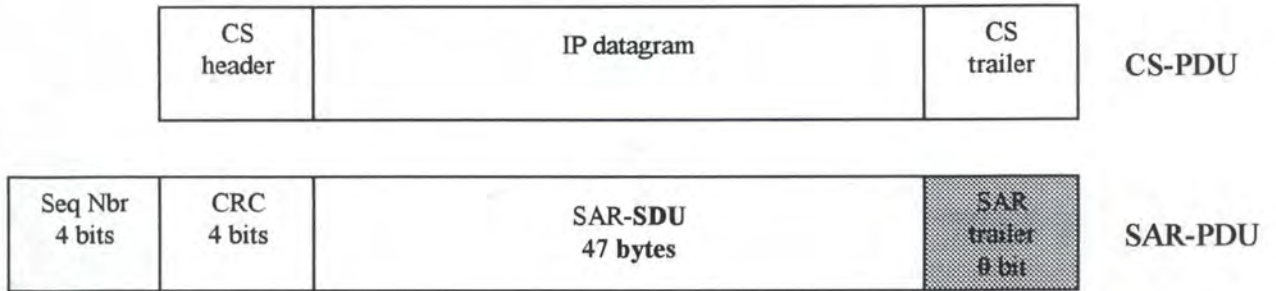
Figure 4-5 : Format des CS-PDU et SAR-PDU pour l’AAL de type 1
