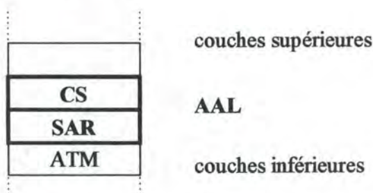
Figure 3-9 : Décomposition de la couche AAL en sous-couches
