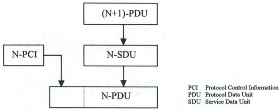
Figure 3-7 : Relations entre les types d'unités de données.
