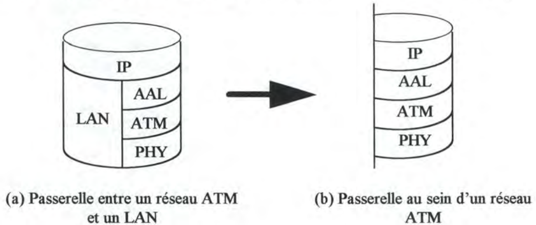
Figure 4-2 : Représentation d'une passerelle dans un réseau ATM
