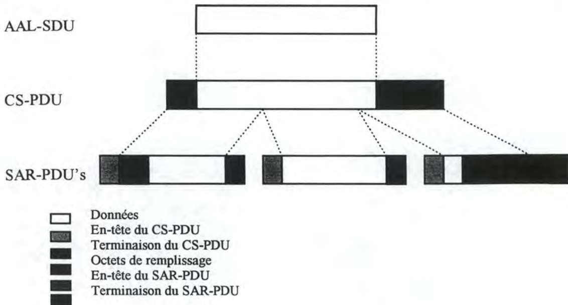
Figure 3-14 : Service en mode message
