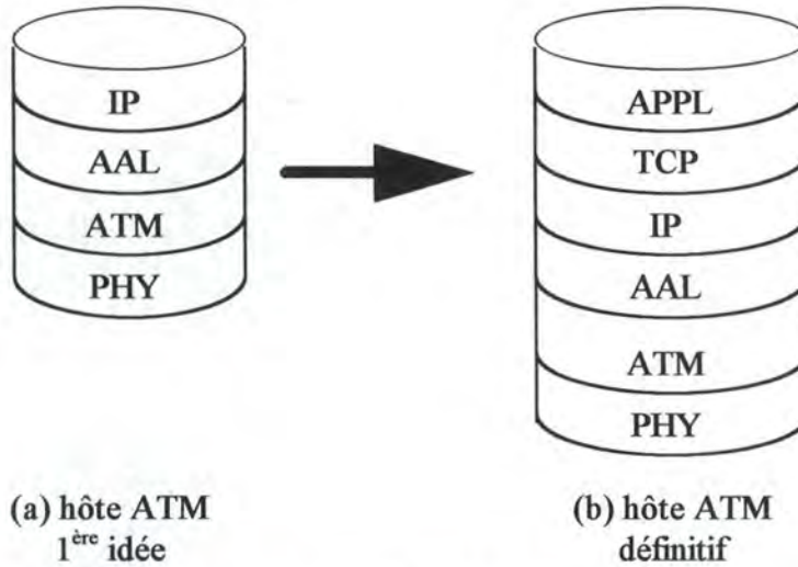
Figure 4-1 : Représentation d'un hôte simple d'un réseau ATM
