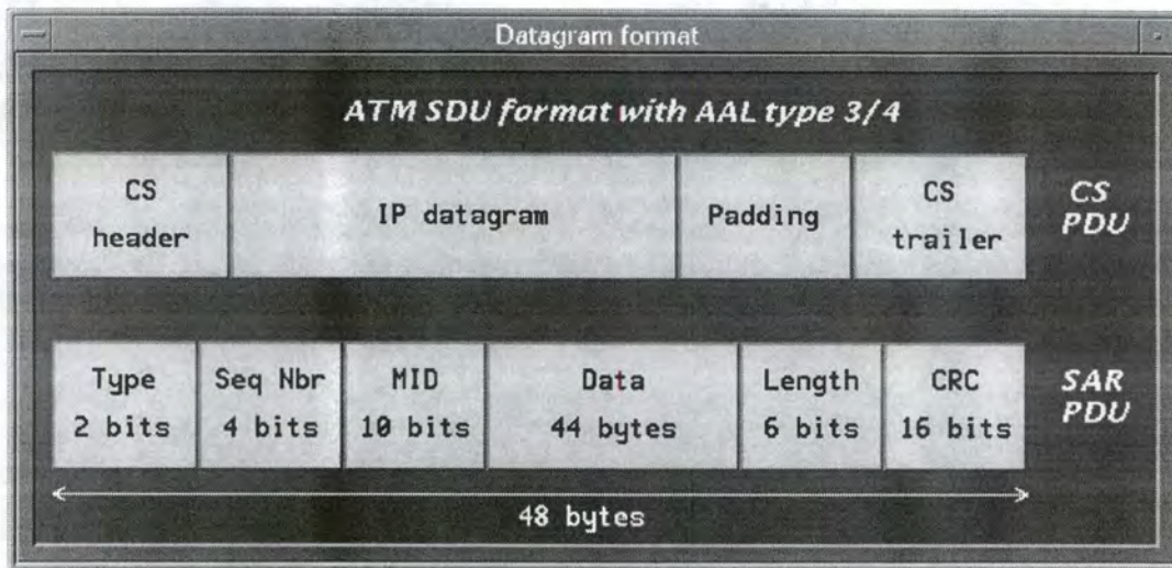
Figure 5-10 :Format des CS-PDU et SAR-PDU pour l'AAL de type 3/4
