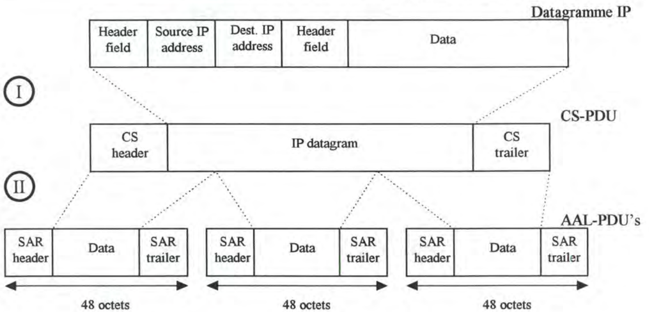
Figure 4-4 : Transformation du datagramme IP en AAL-PDU's
