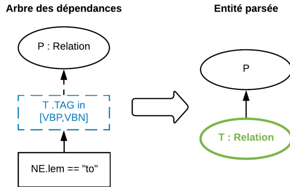
Figure 6.10: Règle de parsing pour la quatrième classe d'AdverbialCausalModifier
