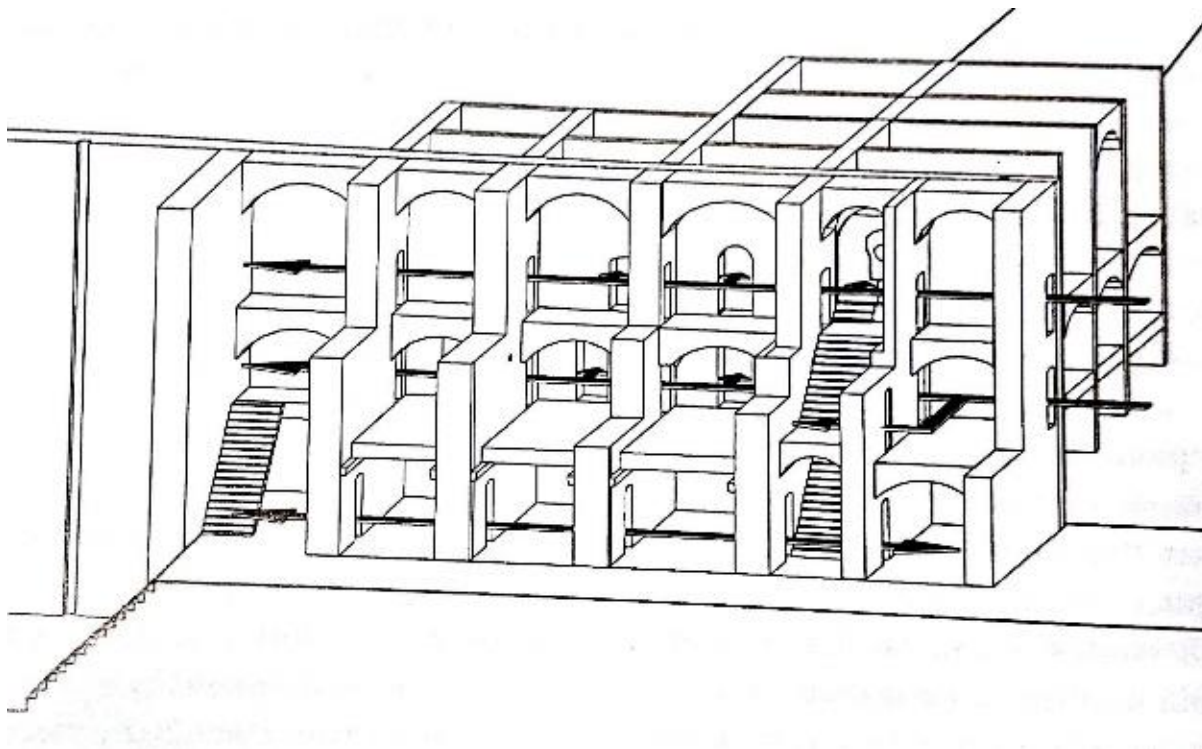
Figure 20 : Rome. Vigna Barberini. Détail de l'angle nord-ouest des soutènements de l'époque d'Hadrien. Accès aux étages supérieurs et circulation interne (VILLEDIEU, F., 1999, p. 763, fig. 7)
