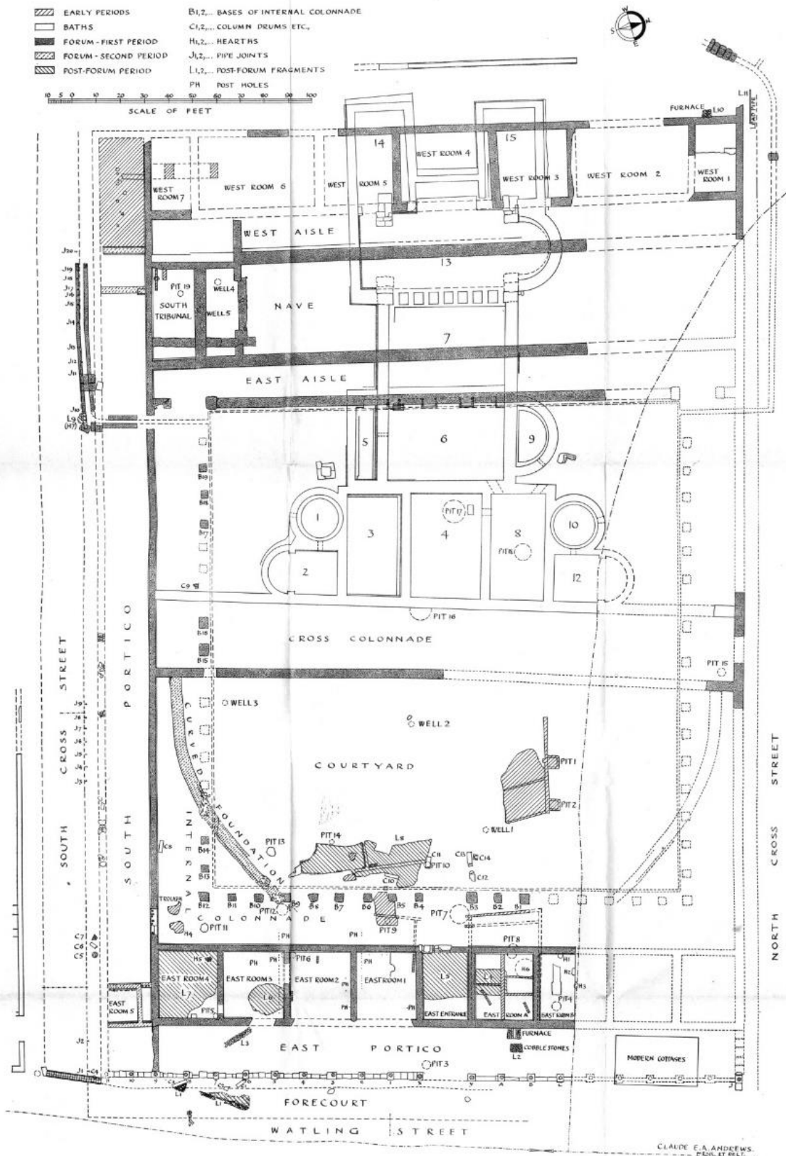
Figure 07. 1 : Viroconium Cornoviorum. Plan d'ensemble du forum (ATKINSON, D., 1942, pl. 1).
