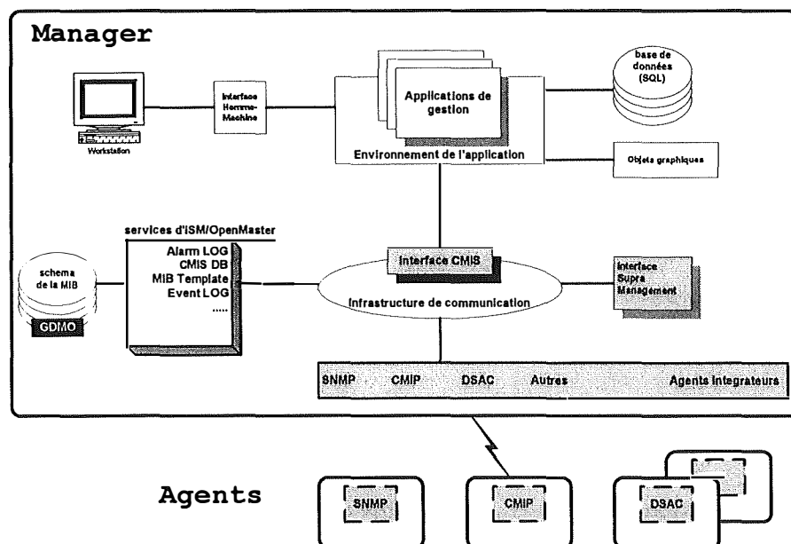
Figure 24 : Une vue unique du modèle de gestion d'ISM/OpenMaster
