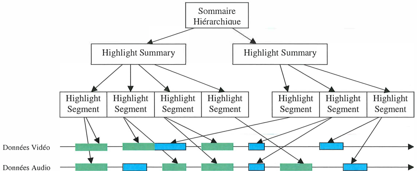
Figure VI-17 : Sommaire hiérarchique
