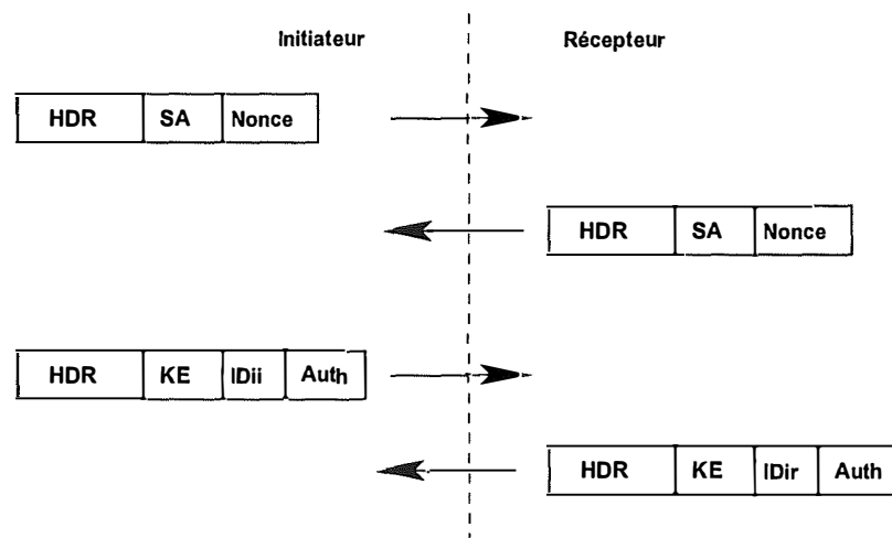
FIG. 1.13 – Echange de base ISAKMP
