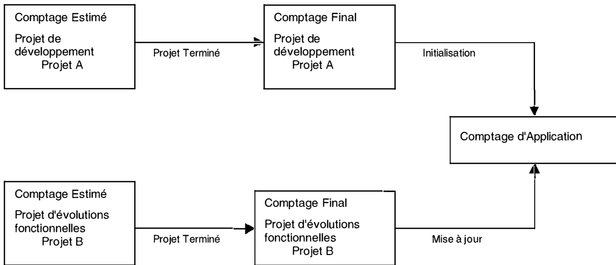
Figure 3: Relation entre les différents types de comptage de la méthode FPA
