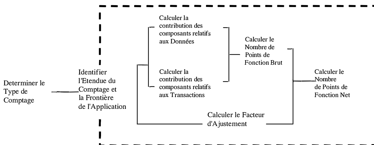
Figure 1 : Étapes de mesure de la méthode de mesure FPA
