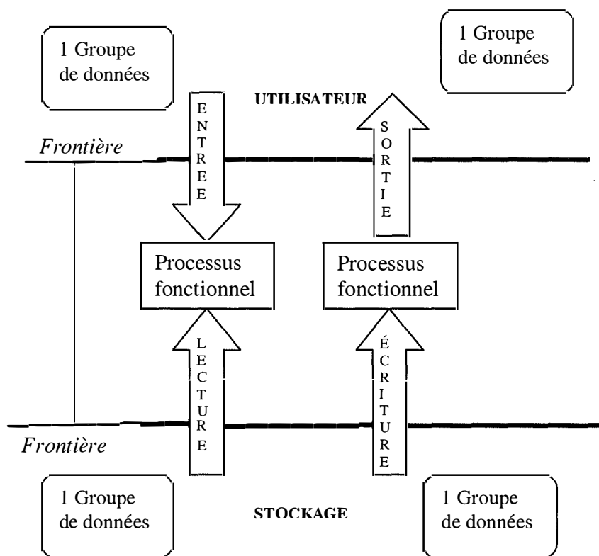
Figure 3-2 : Les quatre types de sous-processus avec leur environnement.
