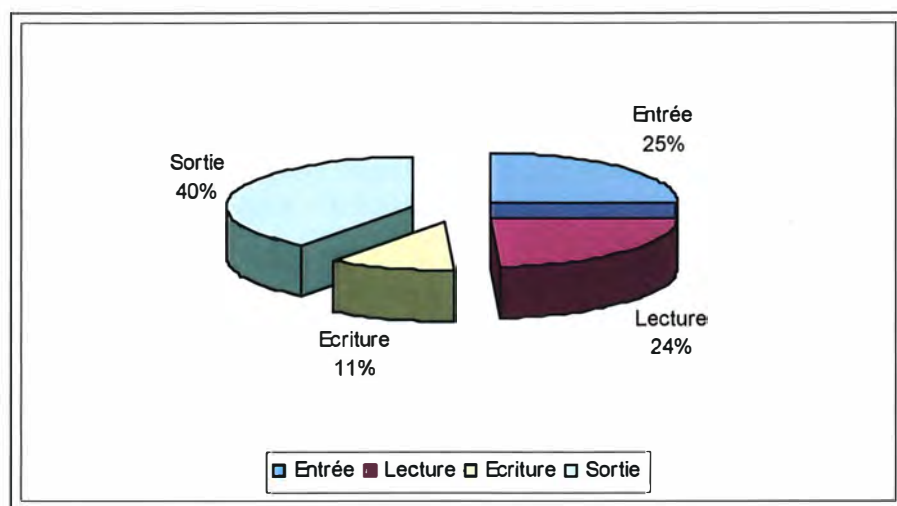
Figure 4-6: Proportion des sous- processus COSMIC-FFP pour l'ensemble des projets mesurés
