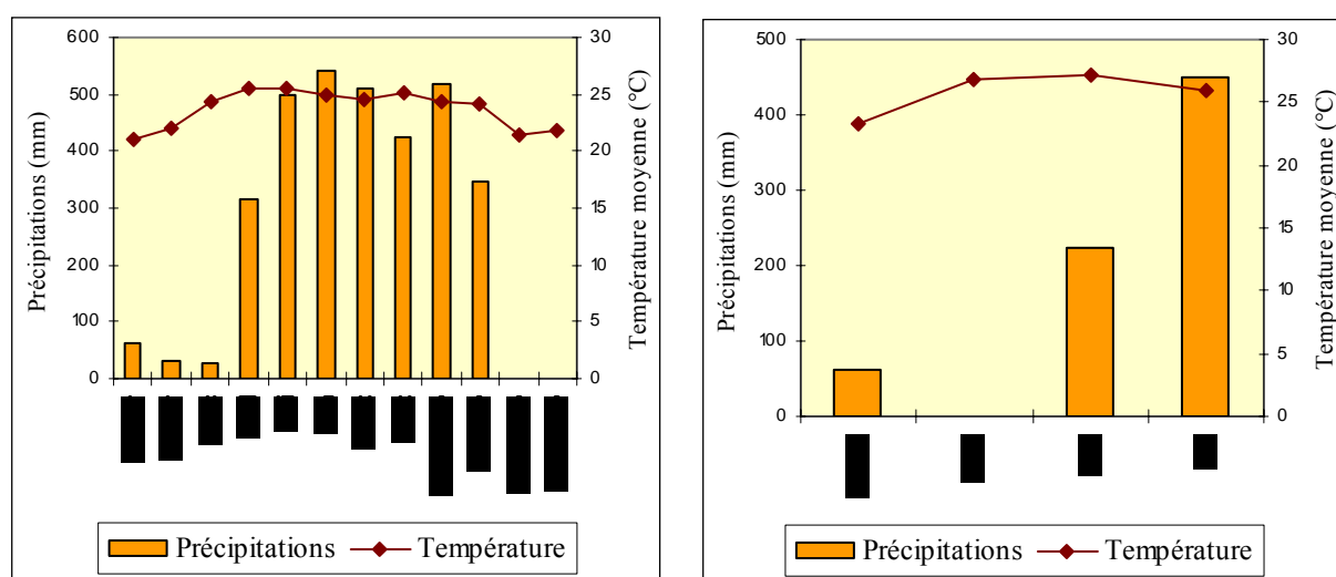
Figure 6 : Climat, températures moyennes et précipitations, au Parc National de Khao Yai en 2000 (Savini, August 2001 - January 2002) et durant les quatre mois de cette étude en 2004.
